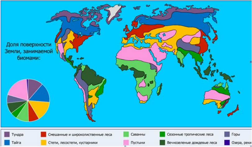
Рис. 10.1. Размещение биомов суши
