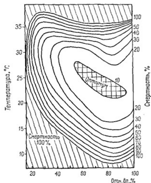
Рис. 3.5. Зависимость смертности куколок яблоневой плодовой жоржки от двух факторов: влажности и температуры
