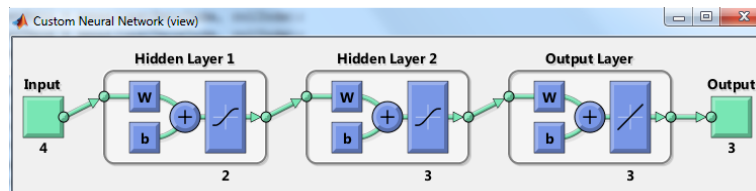
Рисунок 5.9 – Сеть, которая создастся по умолчанию, если в newff() прямо не указать, что нужны функции tansig
