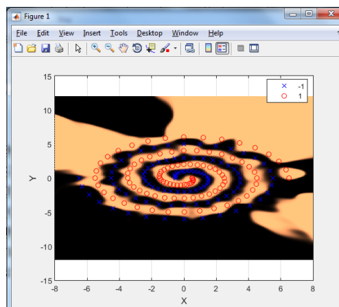
Рисунок 5.17– Поверхность отклика после применения алгоритма trainlm
