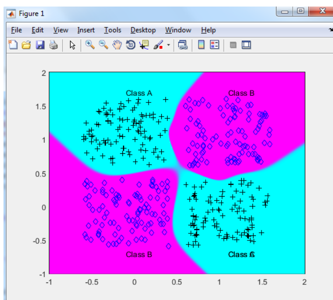
Рисунок 3.28 – Получившаяся граница решения для задачи XOR
