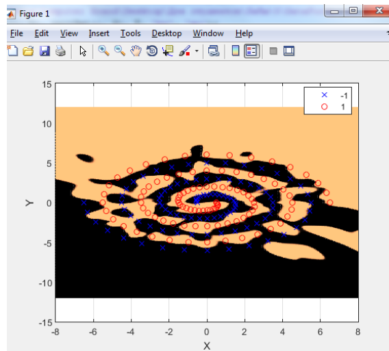
Рисунок 5.18 – Найденное решение с использованием алгоритм trainbfg
