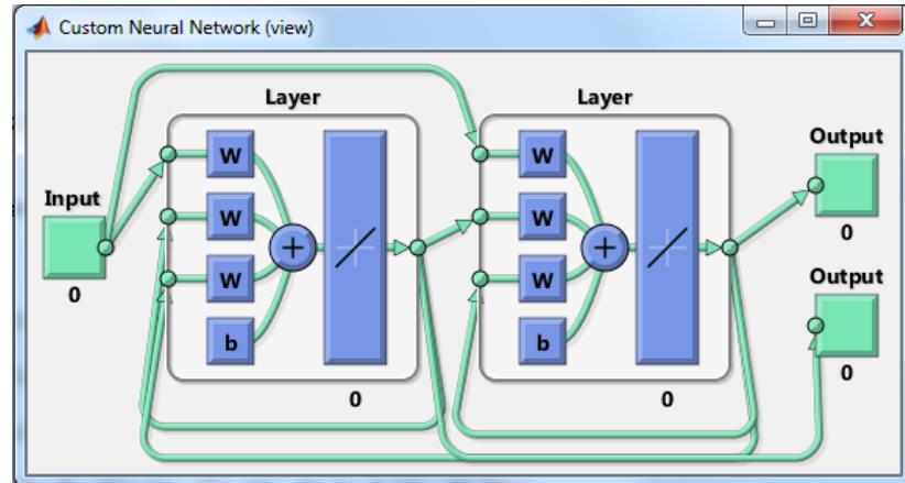
Рисунок 3.7 – Появился второй выход, связанный с первым слоем, а также каждый слой связан с самим собой и второй слой связан с первым (подаёт свои сигналы на вход первого слоя)
