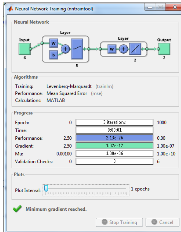
Рисунок 3.10 – Обучение сети
