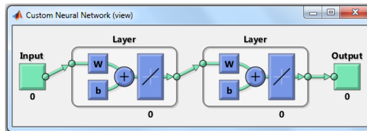
Рисунок 3.5 – Видно, что у второго слоя тоже появилось смещение
