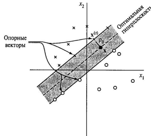
Рисунок 4.2 – Оптимальная гиперплоскость для линейно разделимых образов
