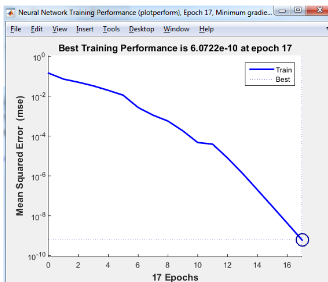
Рисунок 3.30 – Ошибка обучения для сети 2-5-1 Граница
