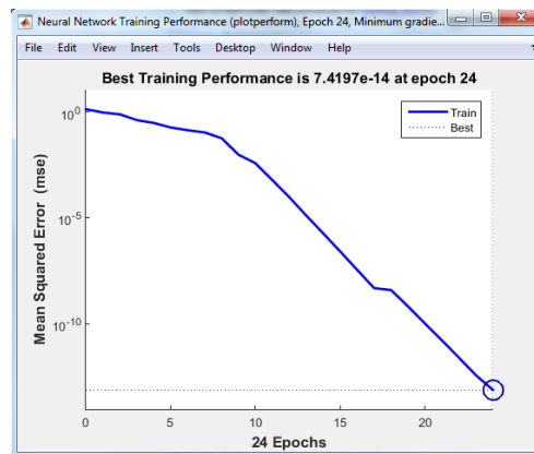
Рисунок 3.25 – Кривая обучения (MSE), лучший показатель меньше 10^{-10} Далее отображаем на новой канве ожидаемый ответ сети, рисунок 3.26.
