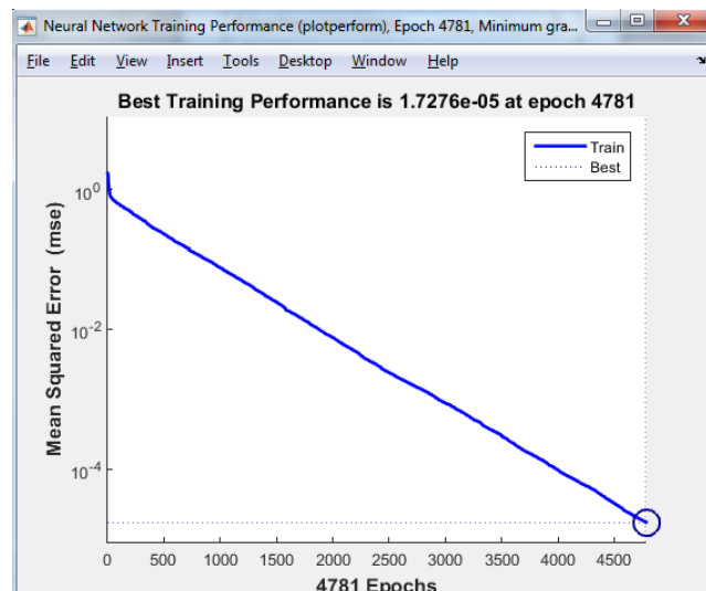
Рисунок 5.21 – Изменение величины ошибки обучения за 5000 эпох
