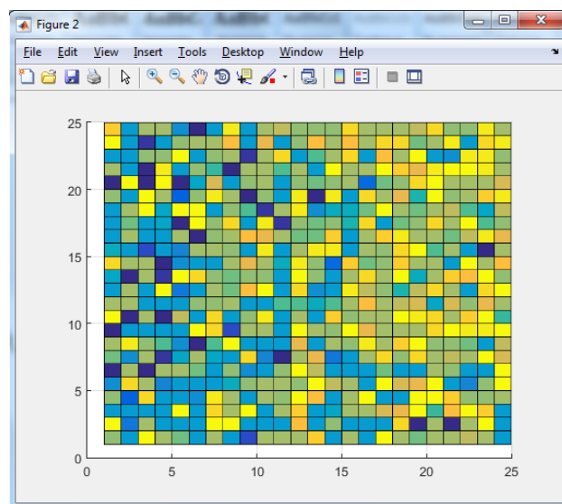
Рисунок 5.11 – Массив valCor
