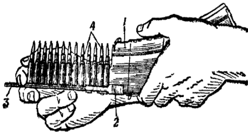
Рис. 63. Снаряжение магазина патронами из обоймы:
