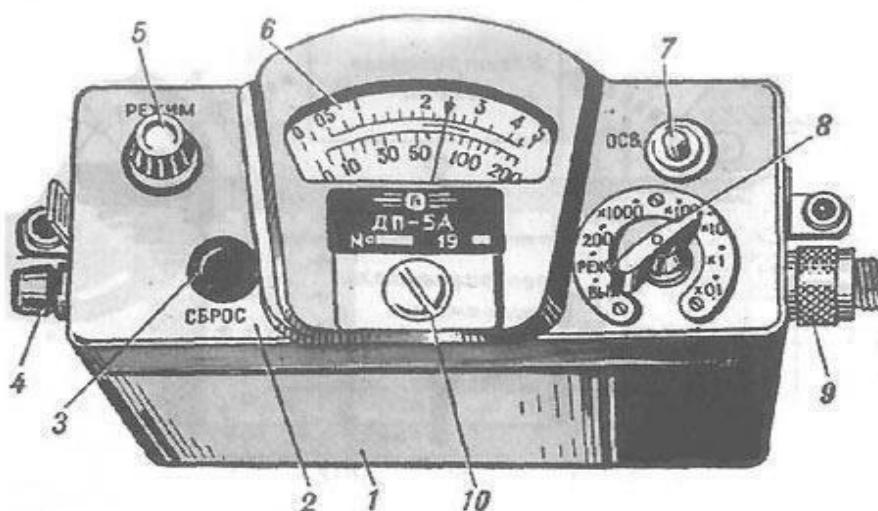
Рисунок 2.7 – Измерительный пульт рентгенометра дозиметра ДП-5 А: 1 — кожух; 2 — панель; 3 — кнопка сброса показаний микроамперметра; 4 — гнездо включения
