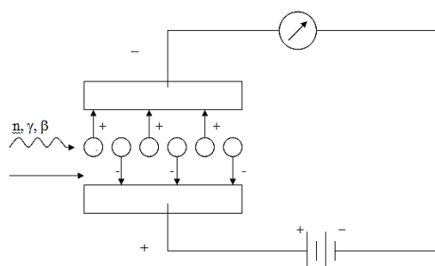
Рисунок 2.3 – Принципиальная схема работы ионизационной камеры
