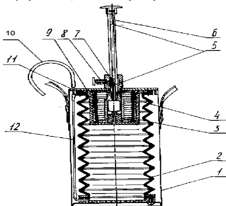
Рис. 12. Газоанализатор УГ-2
