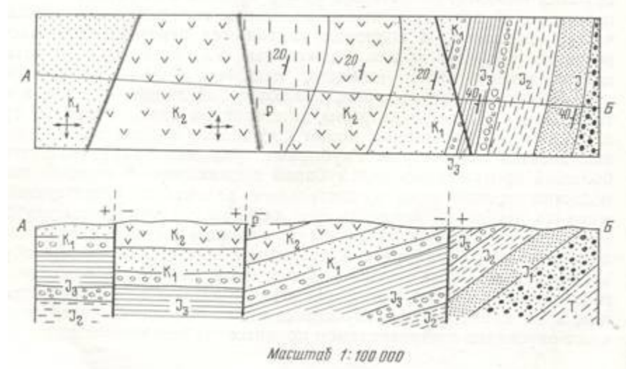
Рис. 28. Построение геологического разреза по геологической карте района, сложенного горизонтально и наклонно залегающими слоями, нарушенными сбросами
