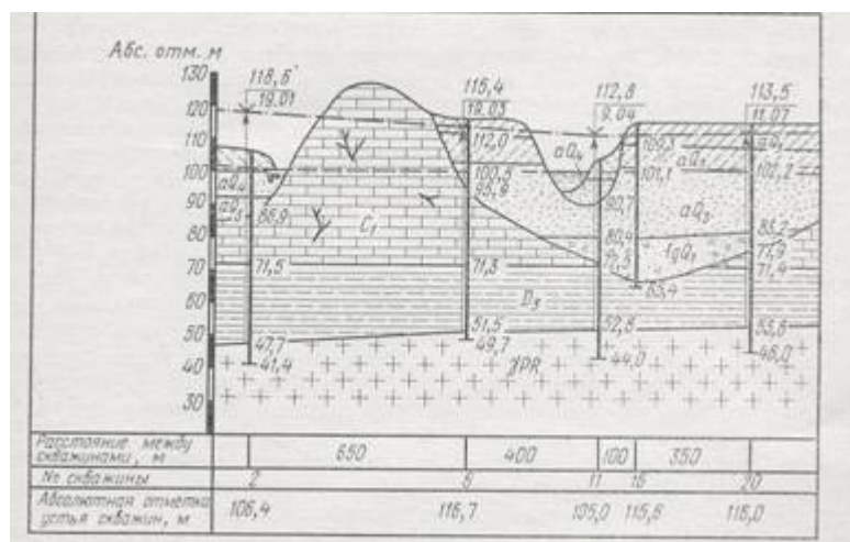
Рис.50. Геологический разрез по линии V-V(на рис. 48)
