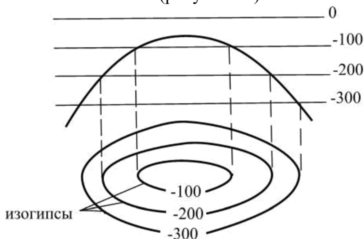
Рисунок 21 Подземный рельеф картируемой поверхности
