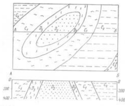
Рис. 27. Построение геологического разреза через антиклинальную складку
