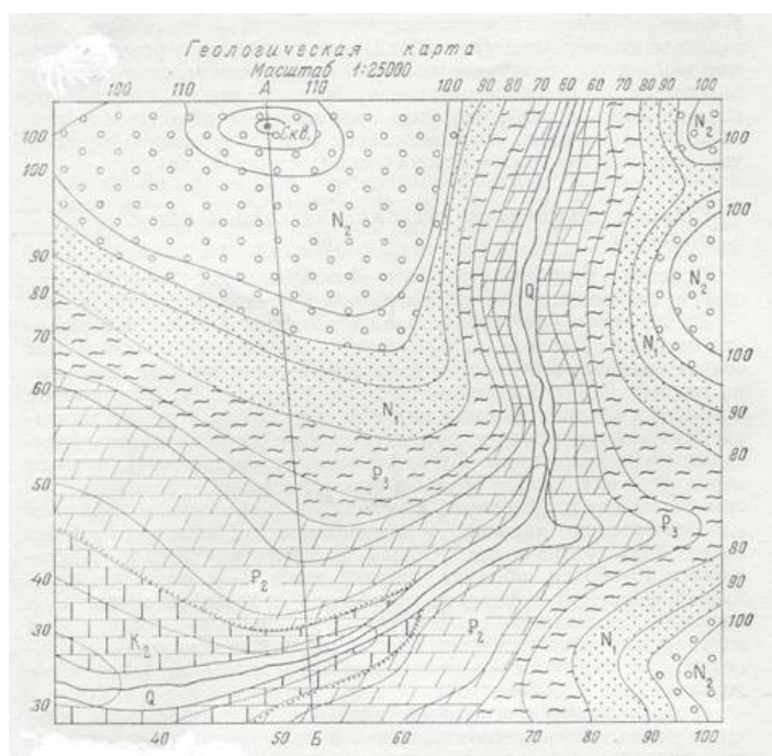
Рис. 32. Геологическая карта участка на топографической основе с горизонтальным залеганием слоев (к зад.2)
