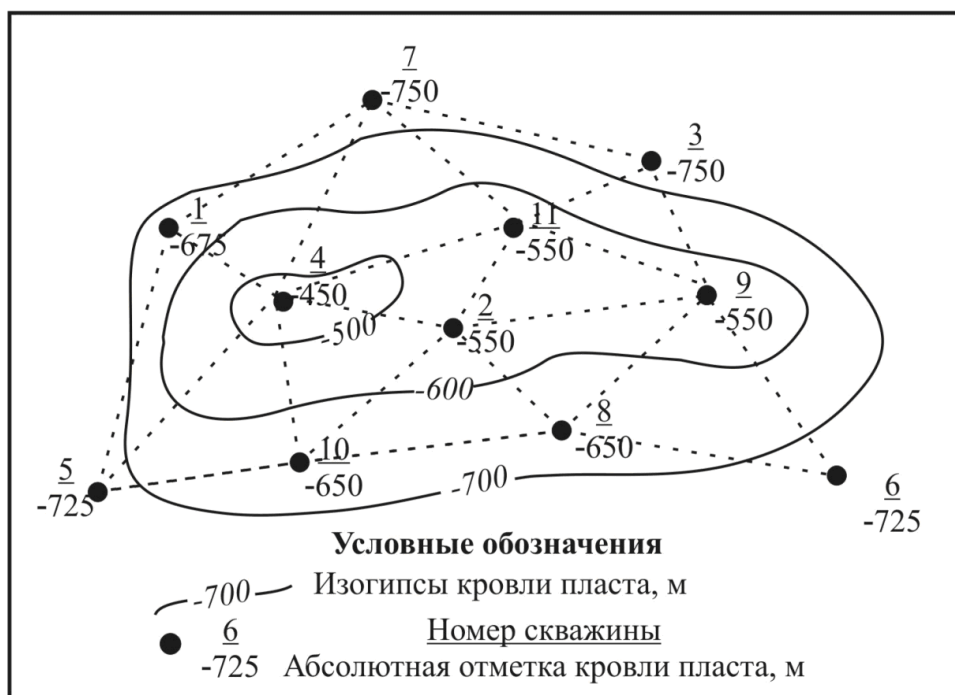
Рисунок 22 Построение структурной карты методом треугольников (по М.А. Жданову)
