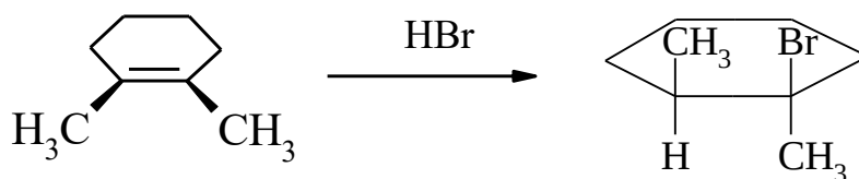
(Z)-1-бром-1,2-диметилциклогексан (рацемат)
