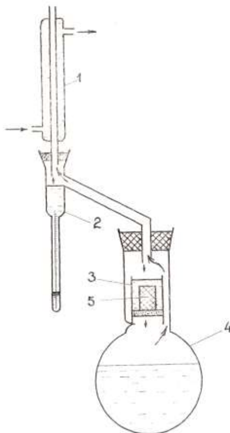
Рис. 7.1. Прибор Закса
