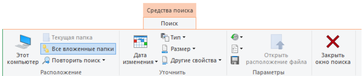
Рис. 42. Средства поиска
