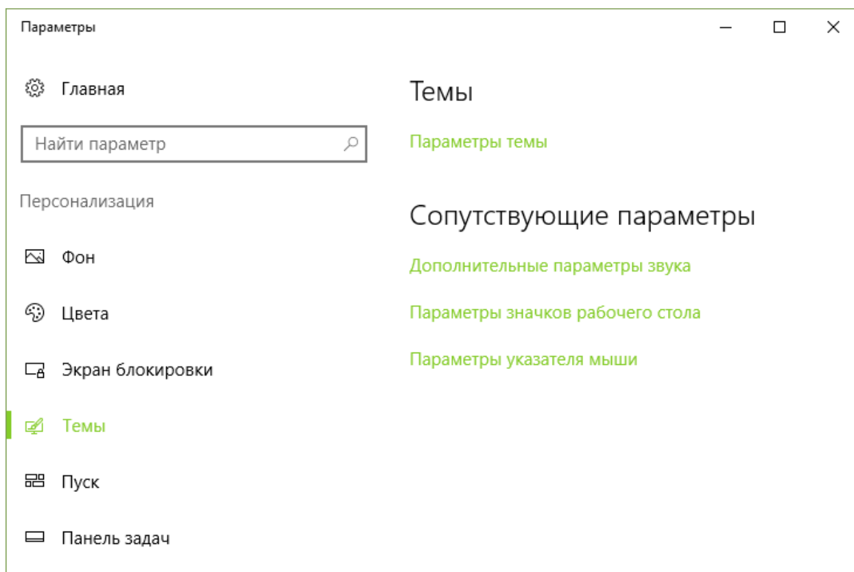
Рис. 16. Меню Темы
