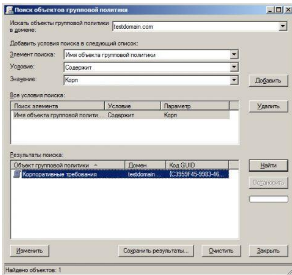
Рис. 11. Результаты поиска
