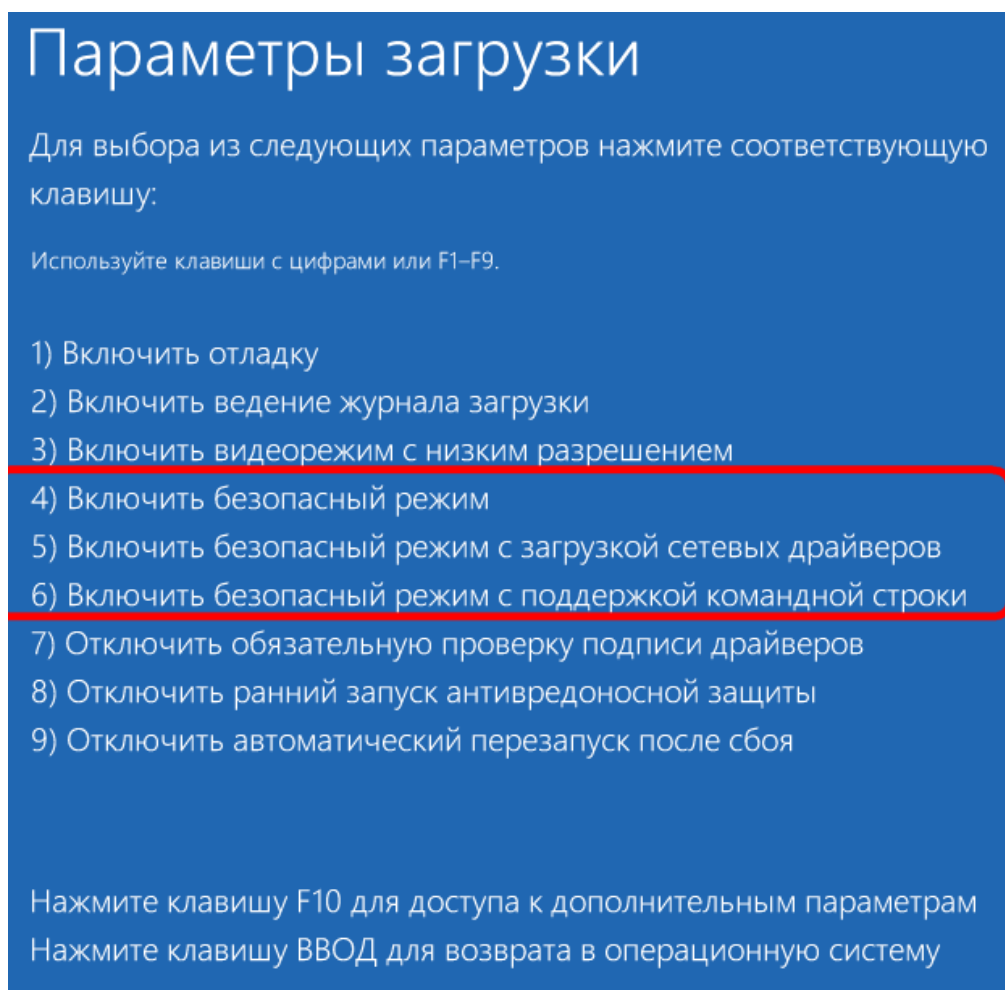
Рис. 9. Параметры загрузки
