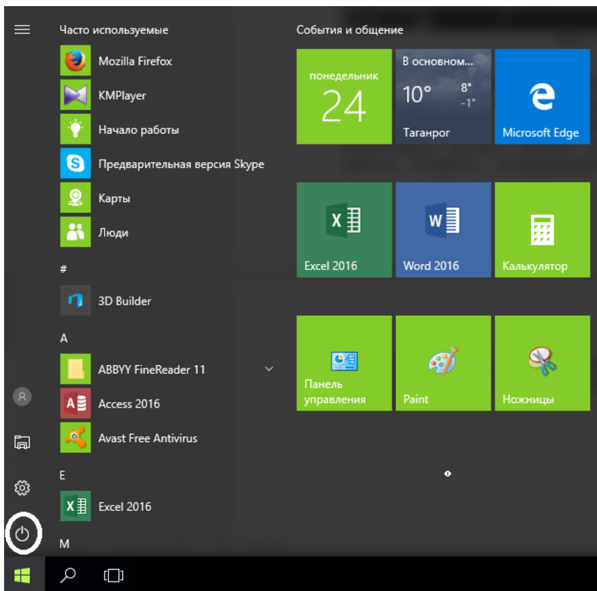
Рис. 2. «Пуск»
