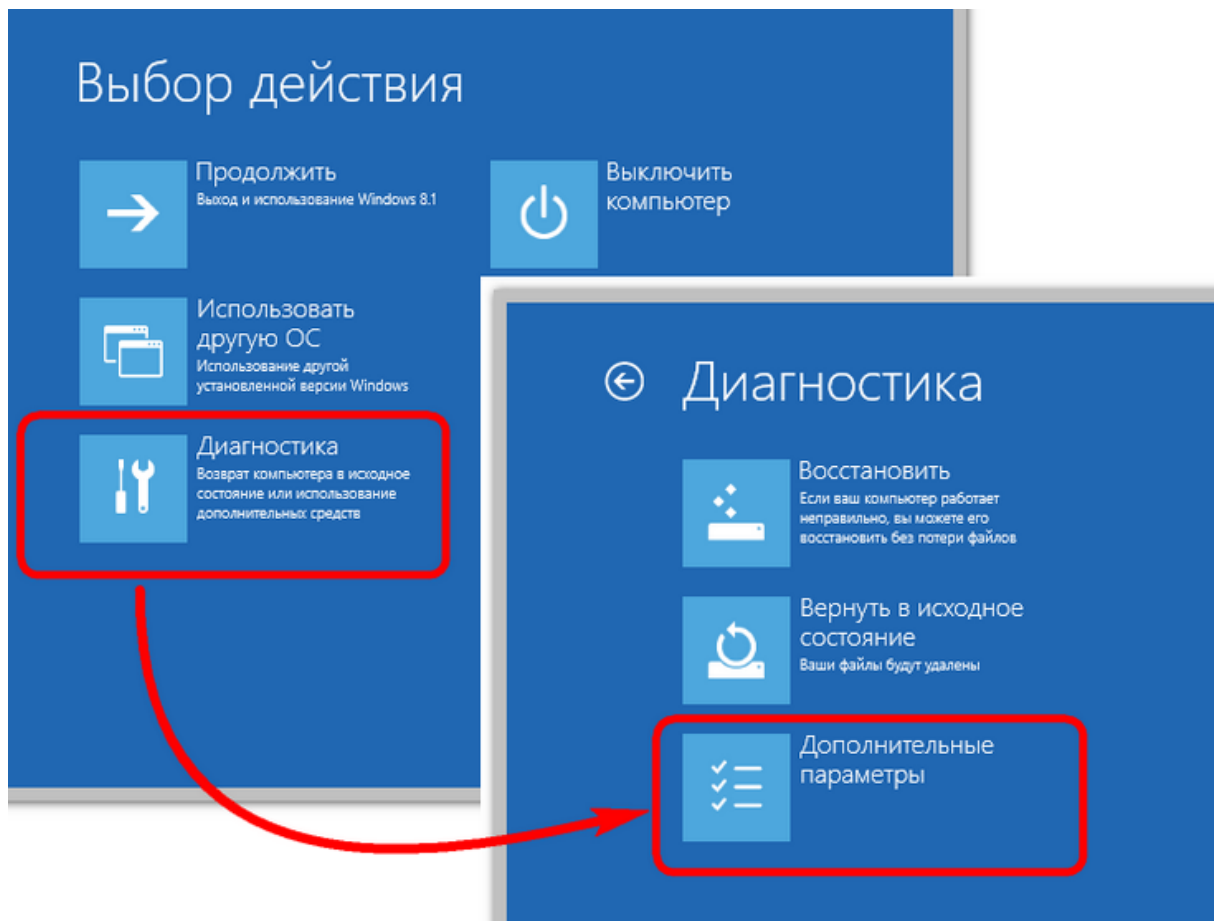
Рис. 7. Раздел Диагностика
