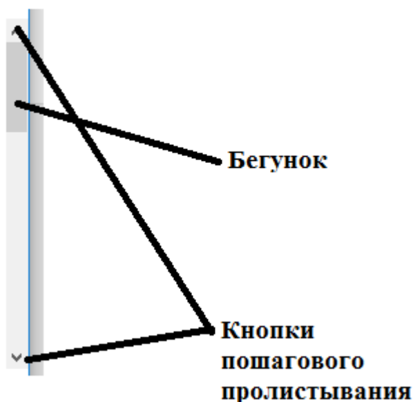
Рис. 25. Линейка прокрутки
