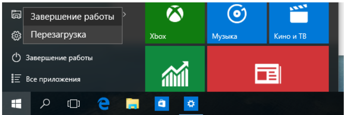
Рис.6. Перезагрузка системы
