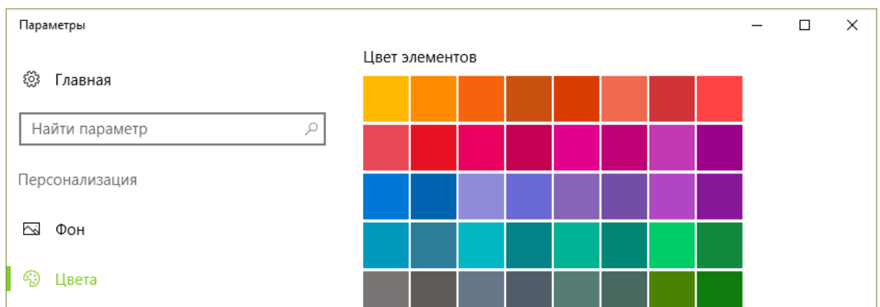
Рис. 13. Меню Цвета
