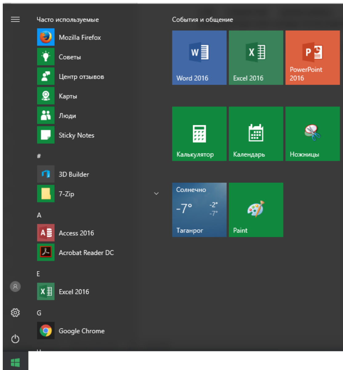
Рис. 43. Меню Пуск
