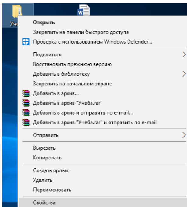
Рис. 21. Меню Свойства
