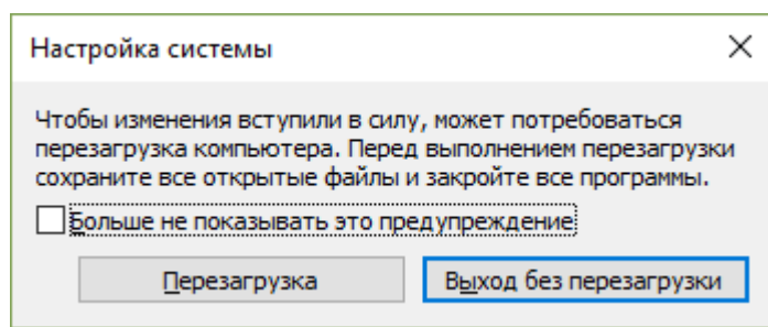
Рис. 5. Настройка системы
