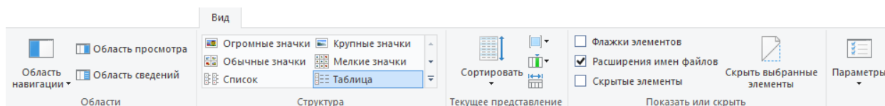
Рис. 26. Меню Вид
