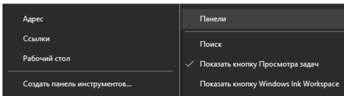
Рис. 33. Меню Панели
