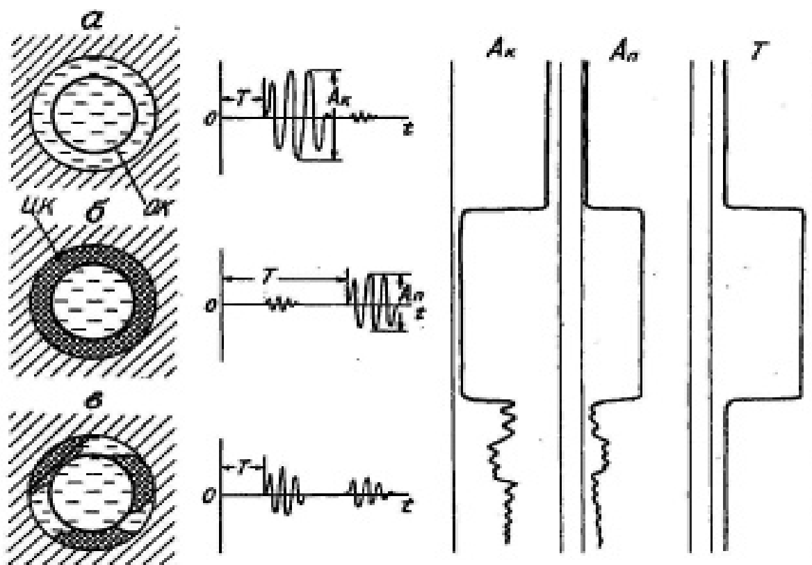
а - при отсутствии цемента в затрубном пространстве; б - при полном заполнении затрубного пространства и хорошем сцеплении цементного камня с обсадной колонной и стенкой скважины; в - при частичном заполнении затрубного пространства цементным камнем Рисунок 6 – Оценки качества цементирования по данным АКЦ
