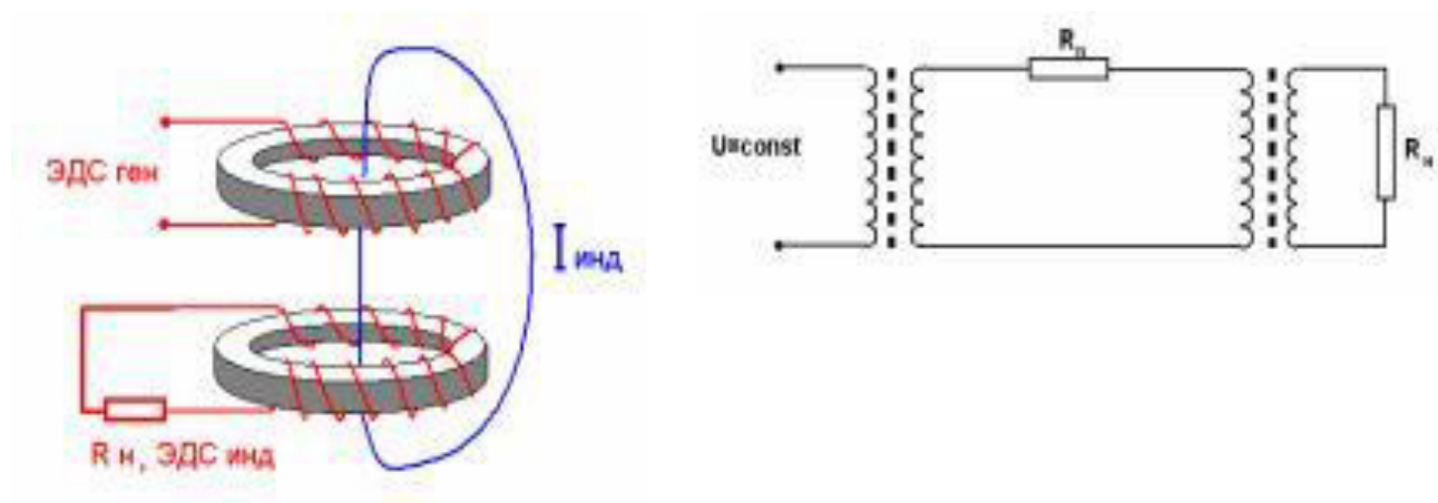
Рисунок 9 – Скважинный индукционный резистивиметр
