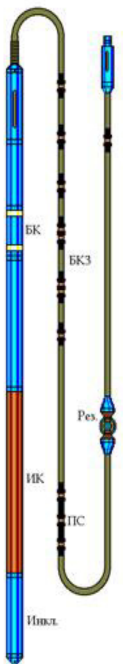
Рисунок 3 – Прибор электрического каротажа
