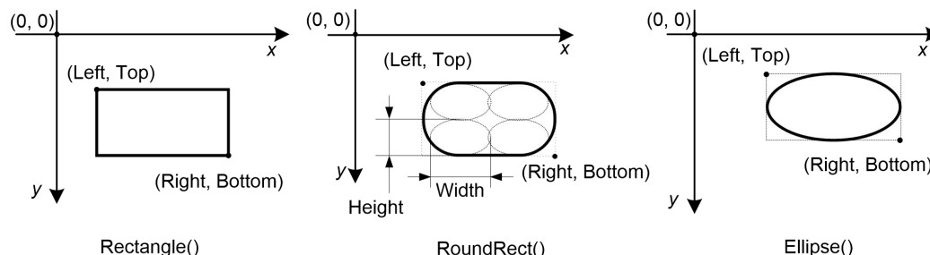
Рис. 9.6. Порядок вывода простейших геометрических фигур
