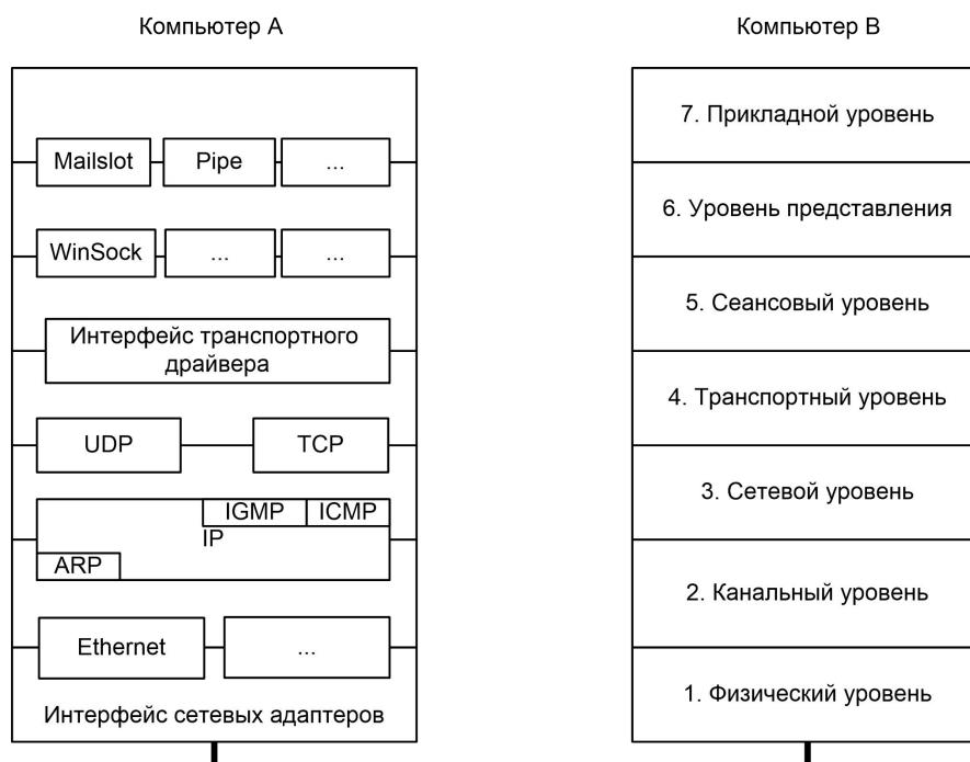
Рис. 6.1. Место сетевых технологий в модели Open System Interconnection
