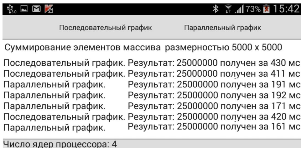
Рис. 3.2. Сравнительные результаты временных затрат на последовательный и параллельный графики
