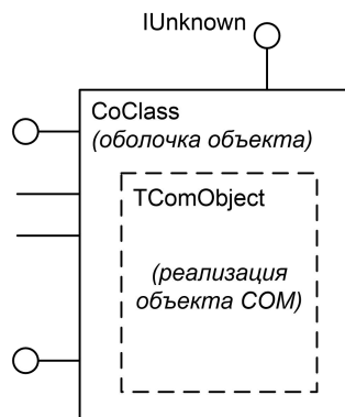
Рис. 8.1. Структура COM-объекта в Delphi
