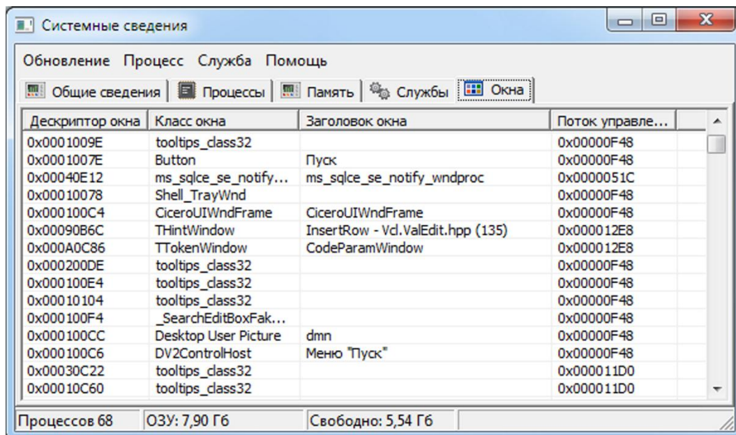
Рис. 5.2. Построение перечня окон с помощью функции EnumWindows()
