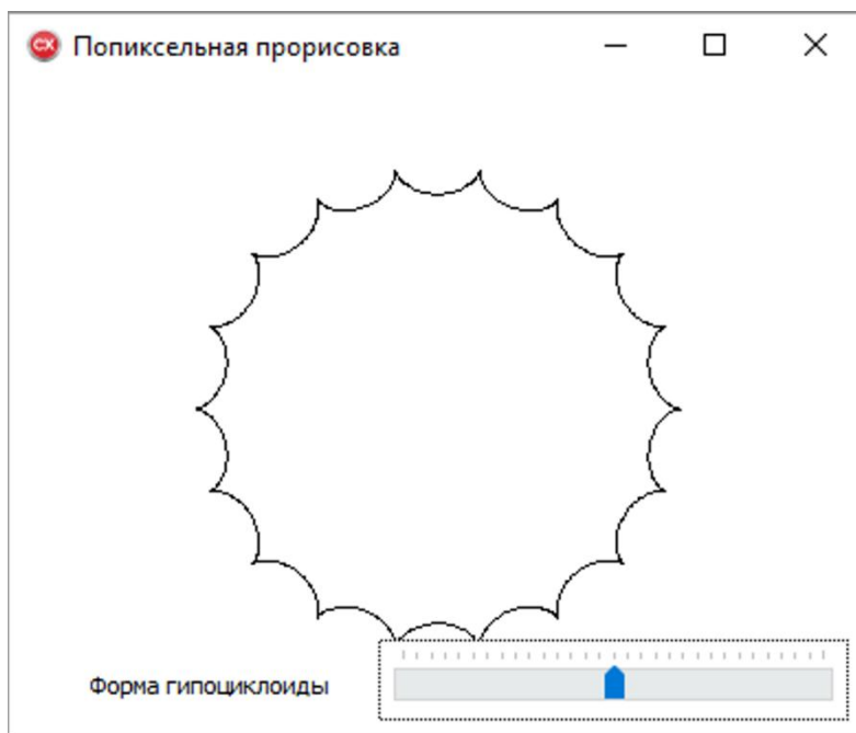
Рис. 9.5. Внешний вид гипоциклоиды
