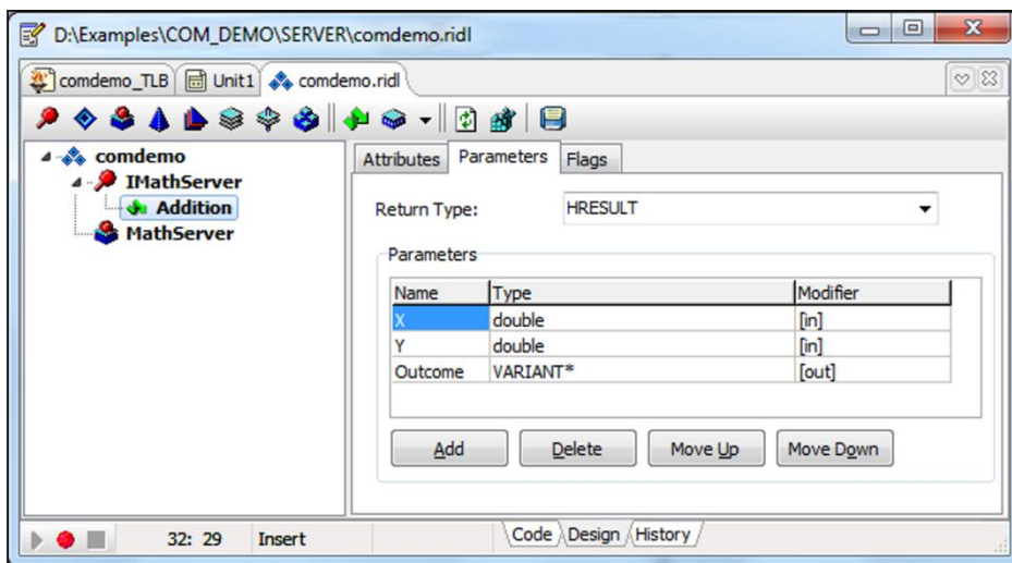
Рис. 8.4. Редактор библиотеки типов с новым методом Addition()
