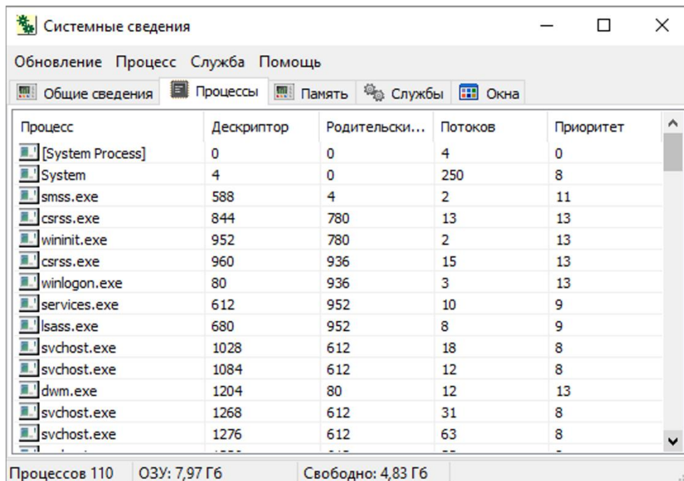
Рис. 2.1. Сбор сведений о процессах Windows
