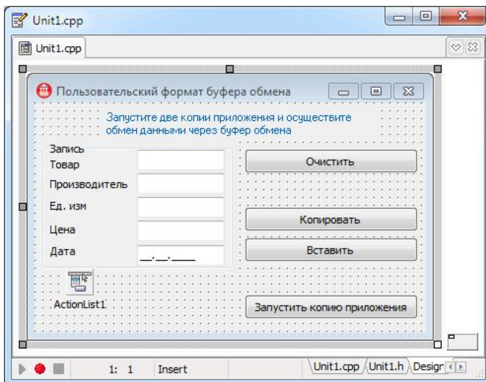
Рис. 5.1. Интерфейс приложения для работы с буфером обмена
