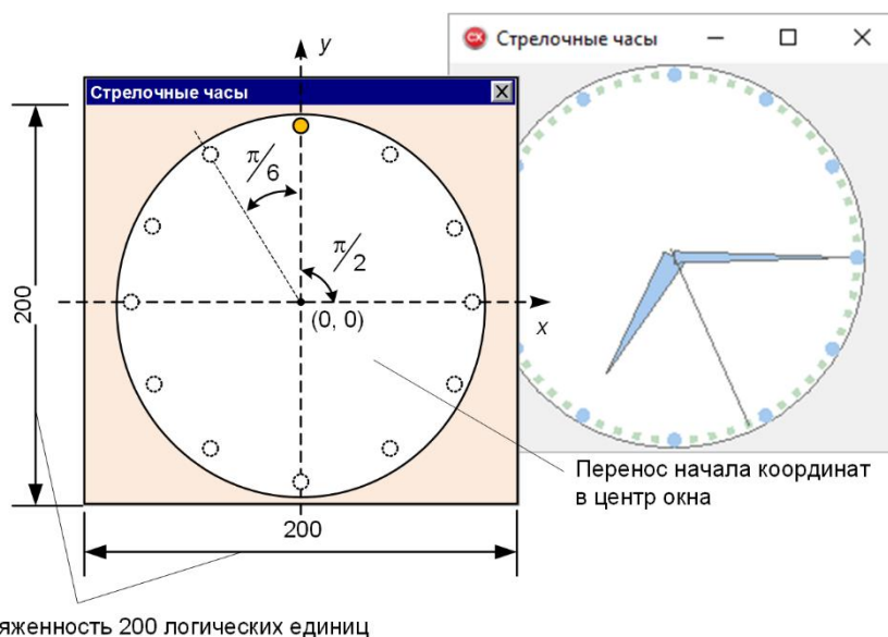
Рис. 9.11. Циферблат стрелочных часов
