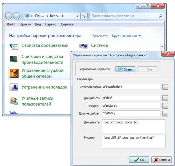
Рис. 7.2. Апплет управления сервисом
