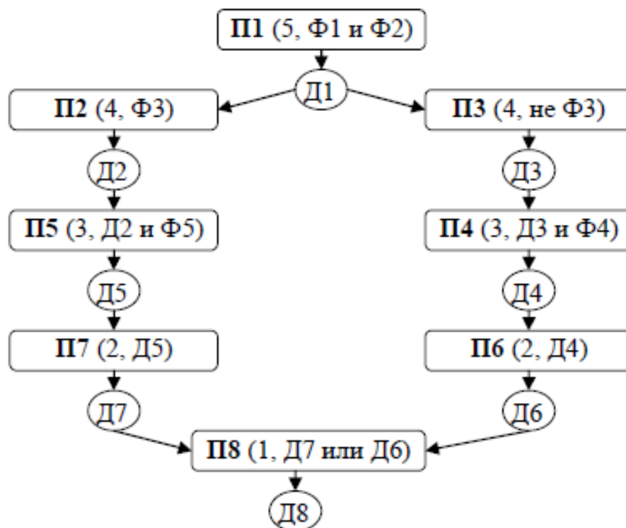
Рис. 1. Схема productions предметной области «Ресторан».
