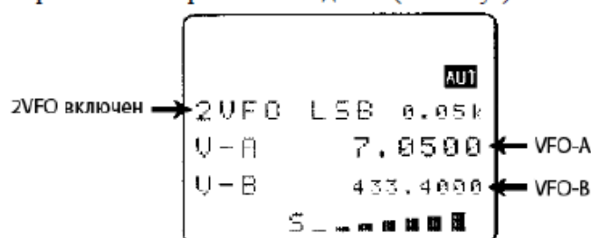
Рис.24. Пример режима 2VFO
