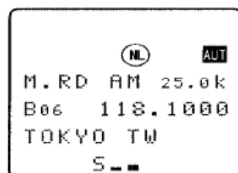
Рис.33. Вид экрана настройки ограничителя шумов
