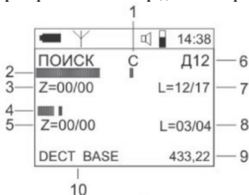
Рис.3. Экран ST107 в режиме «ПОИСК».
