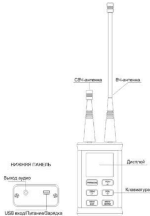
Рис.1 Общий вид ST107
