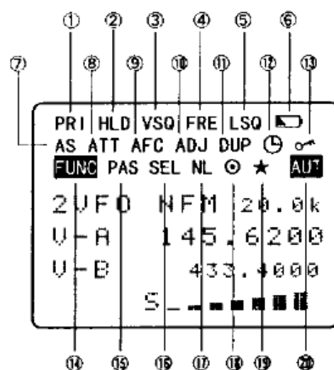
Рис.21. Вид экрана AR8600
