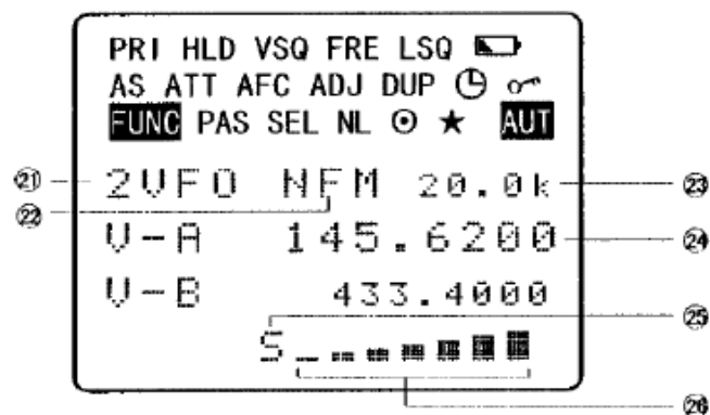
Рис.22. Вид экрана AR8600
