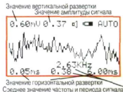
Рис. 9. Описание параметров осциллографа
