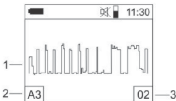
Рис. 6. Экран ST107 в режиме «ОСЦИЛЛОГРАФ».
