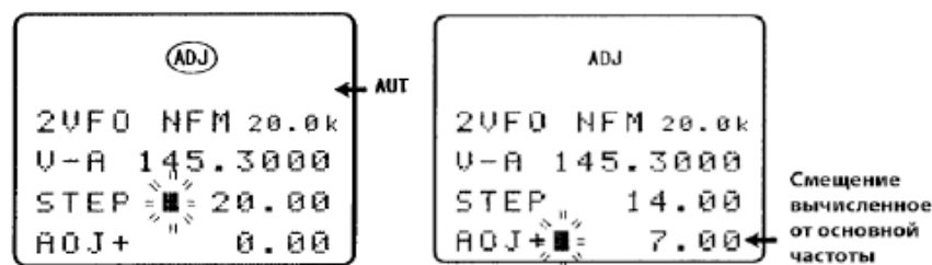
Рис.30. Вид экрана при изменении
