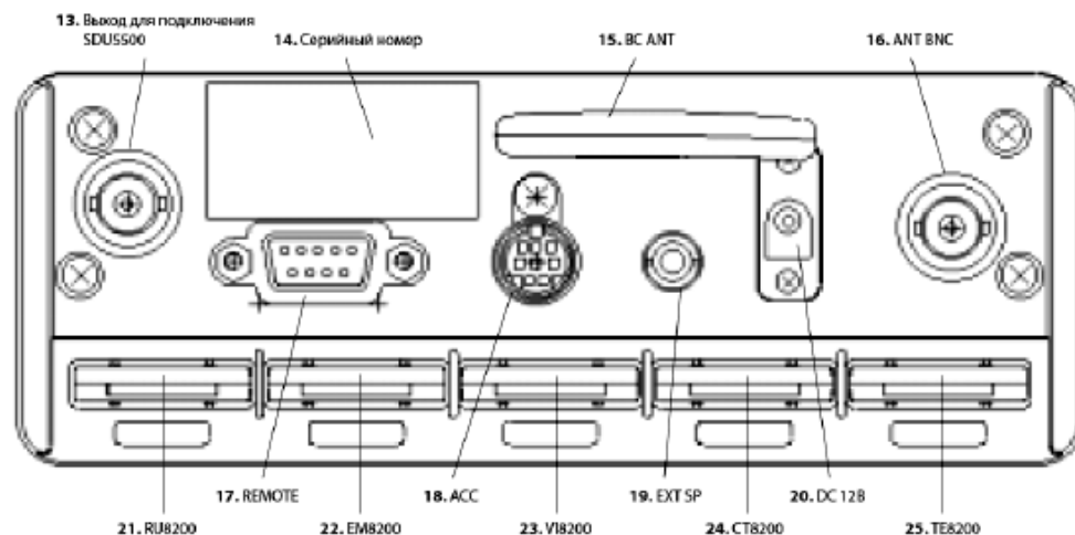
Рис.18. Задняя панель AR8600
