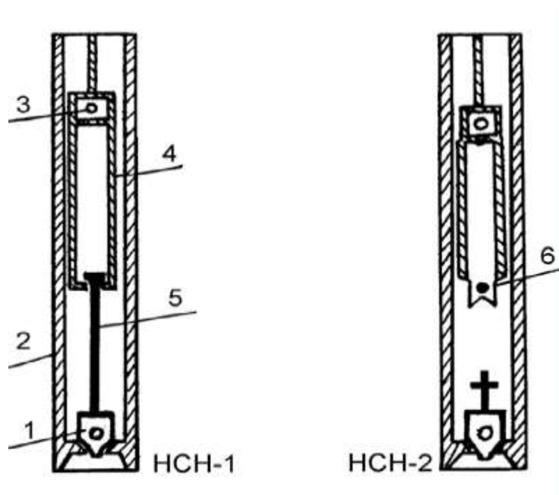
Рис. 15. Невставные скважинные насосы:
