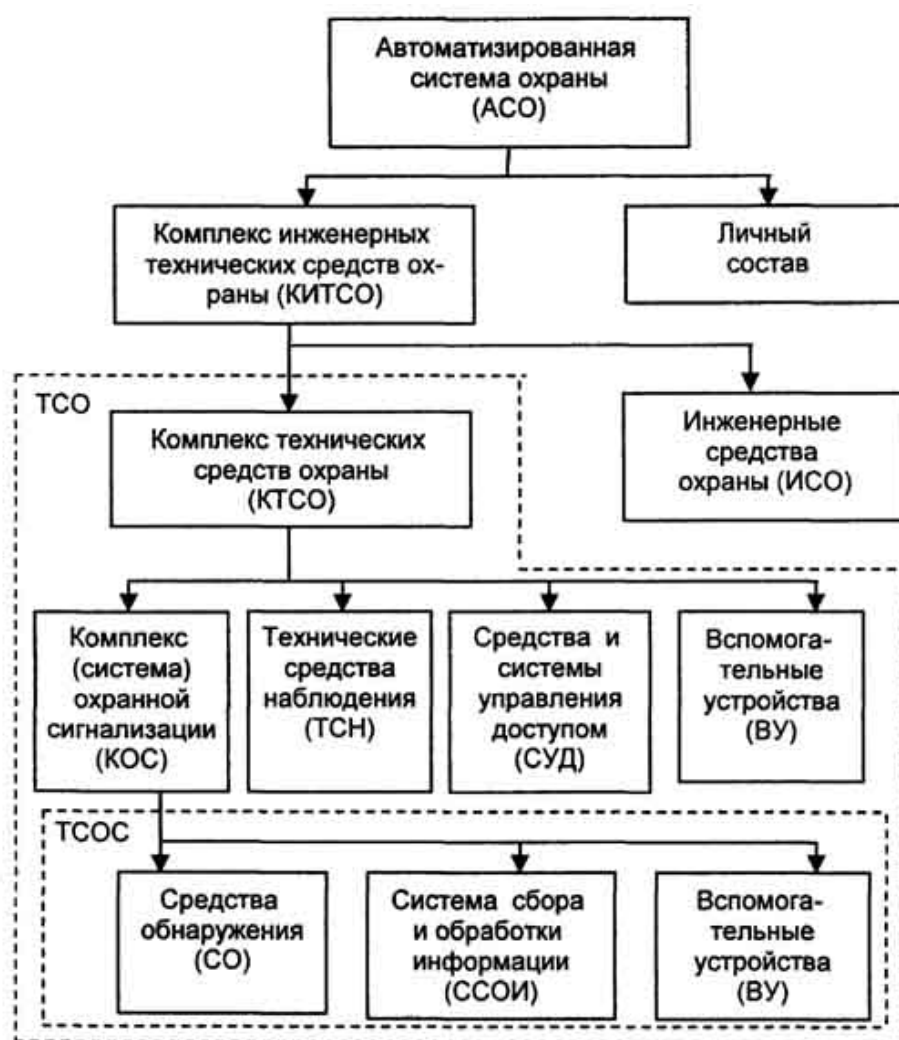
Рис. 1. Структура автоматизированной системы охраны
