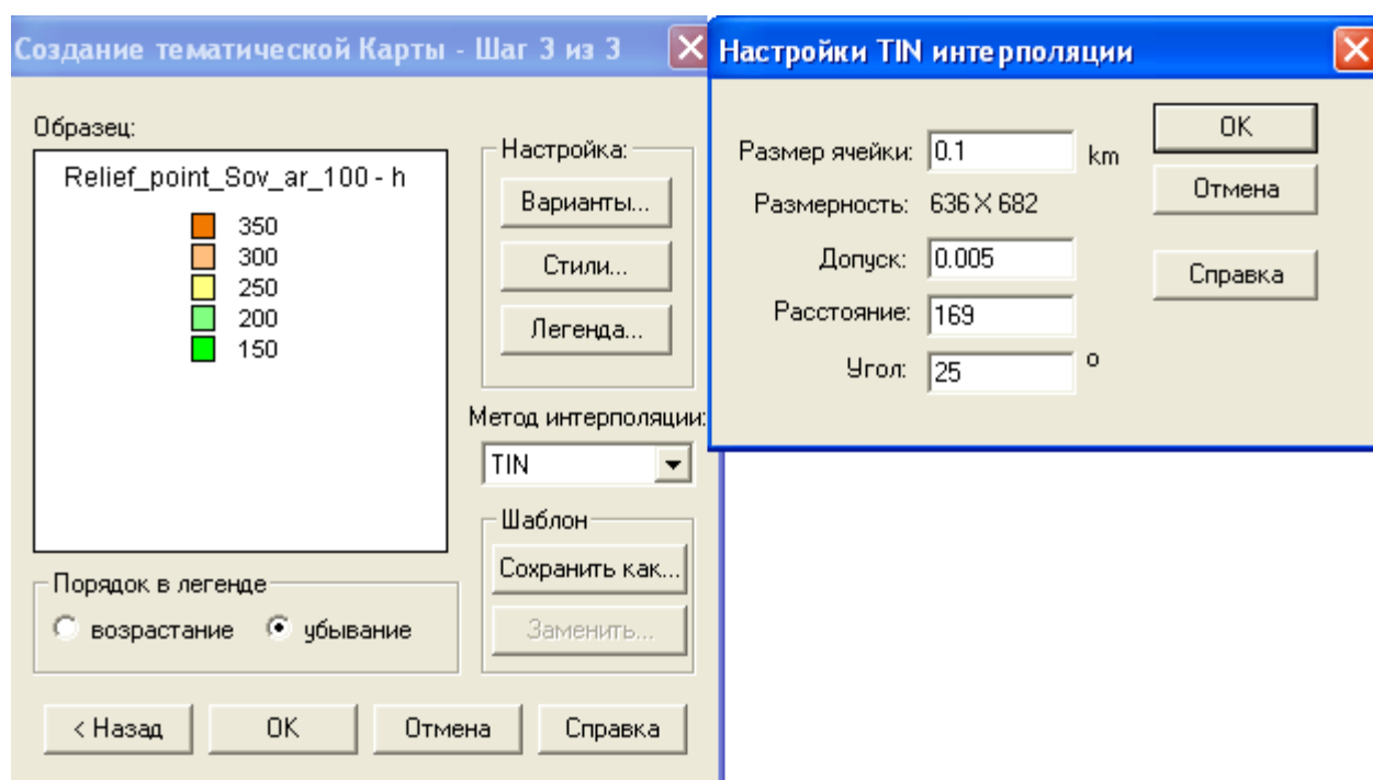
Рис. 19. Окна <Создание тематической карты (поверхности)– Шаг 3 из 3> и <Настройка TIN интерполяции>.
