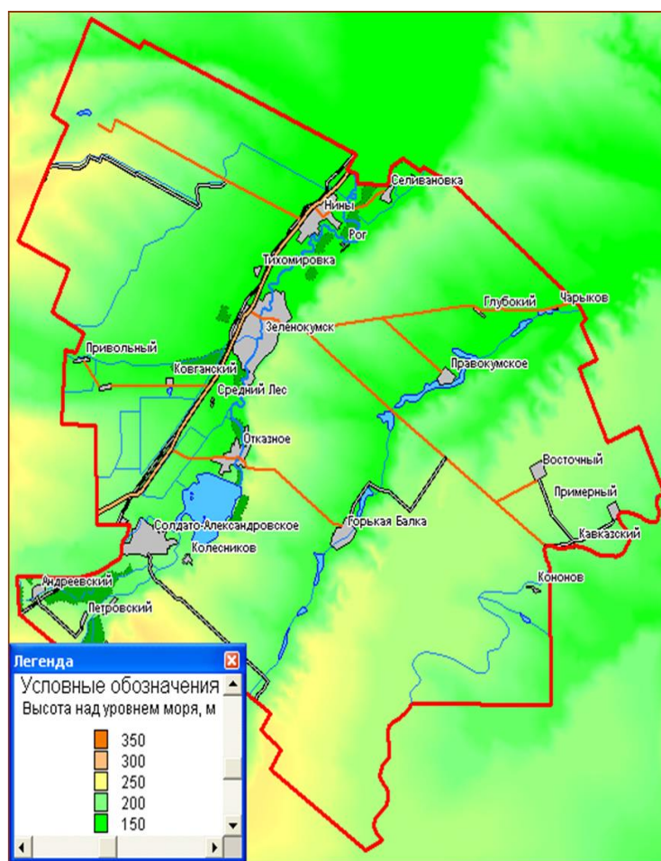
Рис. 21. Результат построения поверхности с наложенной на нее ЦКО.
