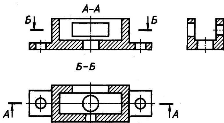
Рис. 6.7. Обозначение разрез
