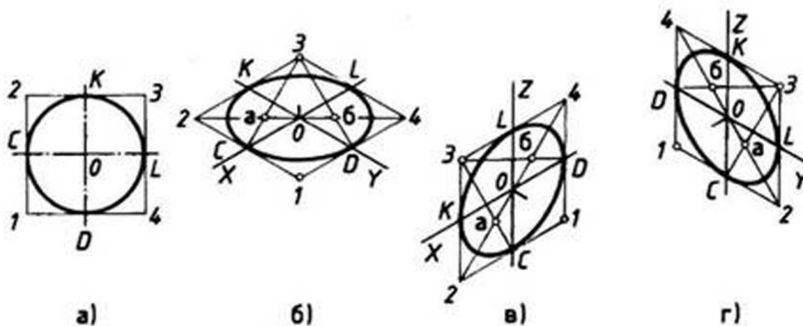
Рис. 5.7. Прямоугольная и изометрические проекции круга
