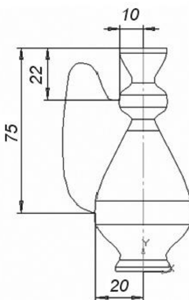
Рис. 8.16. Сечение объекта
