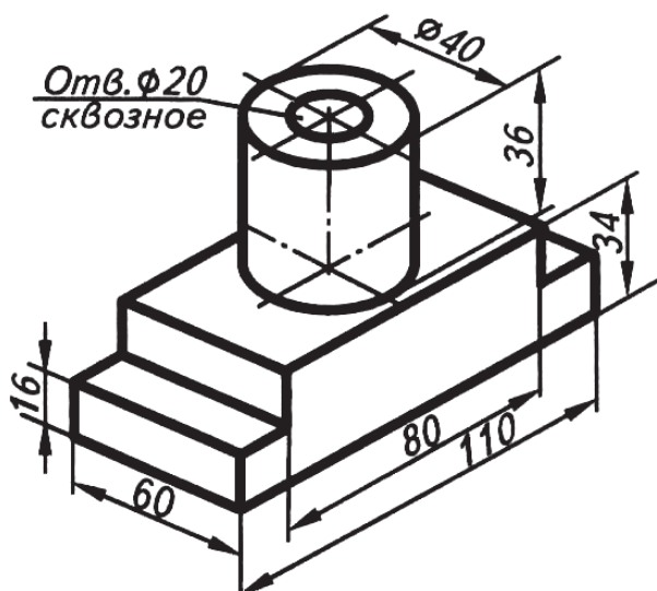
Рис. 7.3. Построение детали
