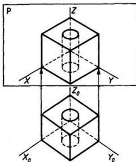
Рис. 5.1. Получение аксонометрической (прямоугольной изометрической) проекции
