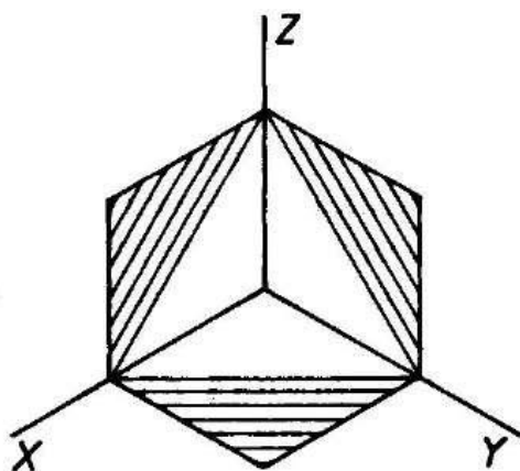
Рис. 6.11. Нанесение штриховки в изометрической проекции.
