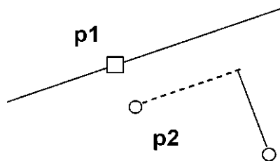
Рис. 1.9. Построение отрезка, перпендикулярного заданной прямой
