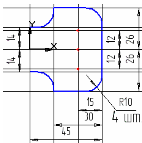
Рис. 3.5. Выполнение скругления
