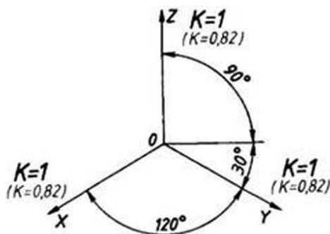
Рис. 5.3. Положение осей и коэффициенты искажения изометрической проекции
