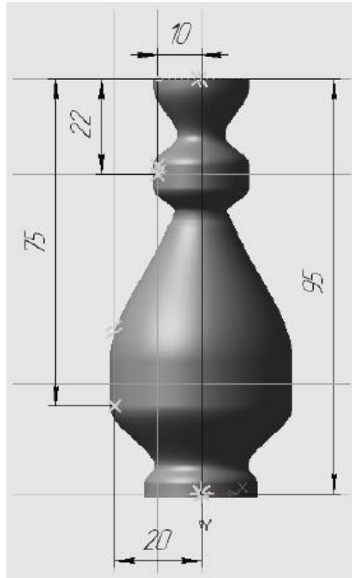
Рис. 8.18. Созданный объект с нанесенными размерами
