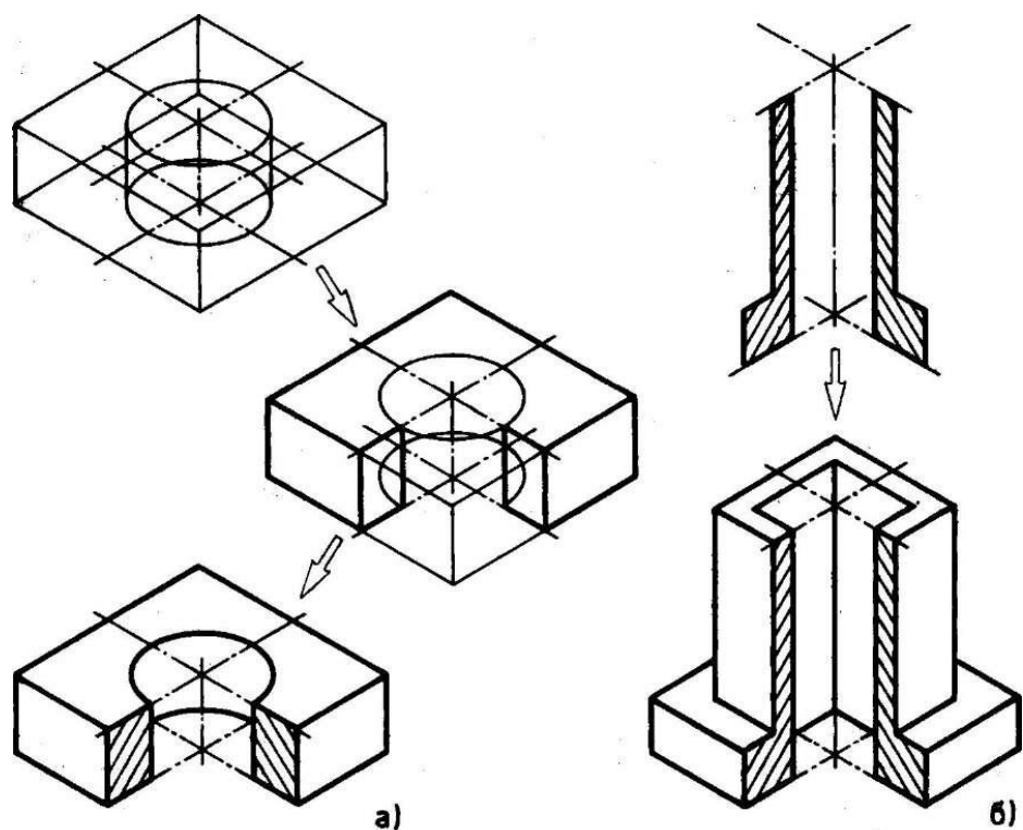
Рис. 6.12. Построение разреза в аксонометрии
