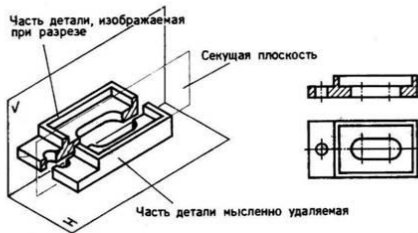
Рис. 6.4. Фронтальный разрез
