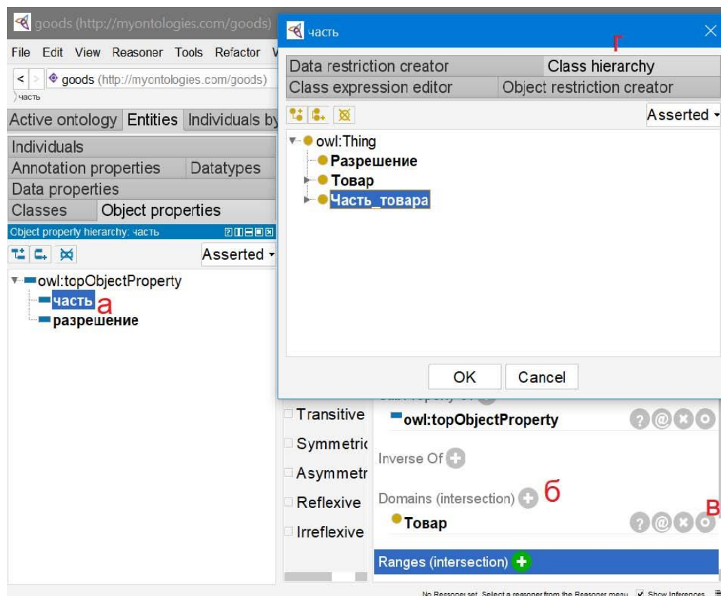
Рисунок 9 Задание информации о Object Property в системе Protégé (а – выделенное свойство «часть», б – кнопка добавления новой области определения, в – кнопка редактирования существующей области определения, г – активная вкладка иерархии классов при задании области определения свойства)
