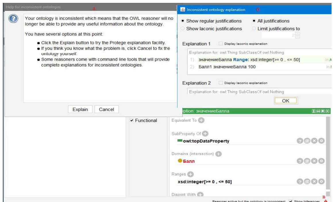
Рисунок 17 Пример ошибки при запуске механизма рассуждений (а – сообщение о проблемах в онтологии с предложением объяснения; б – окно объяснений; в – индикатор ошибок в логах системы)
