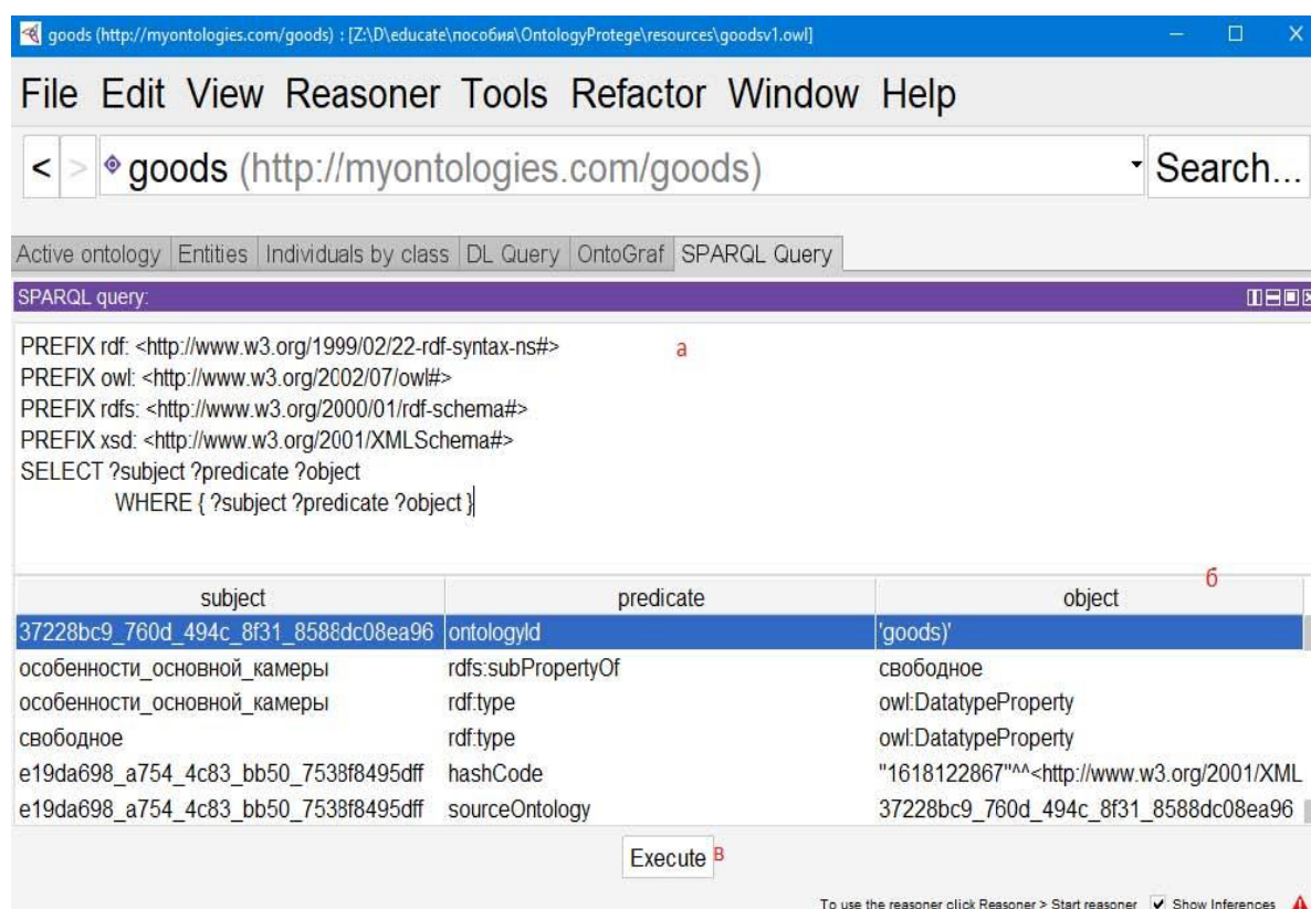
Рисунок 23 Вкладка «SPARQL Query» в системе Protégé (а – поле ввода запроса; б – результаты запроса; в – кнопка выполнения запроса)
