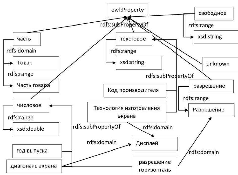
Рисунок 3 Фрагмент графа, описывающего свойства в рамках описания смартфонов
