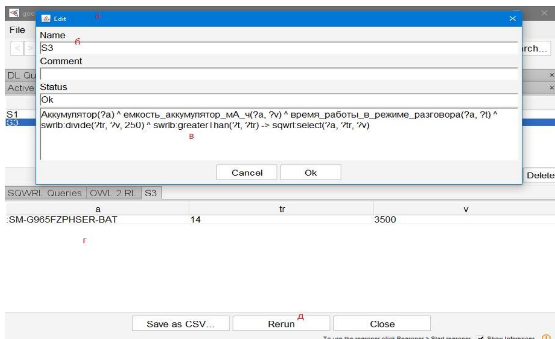
Рисунок 25 вкладка SQWRL в системе Protégé (а – окно редактирования правила; б – имя правила; в – тело правила; г – результаты выполнения правила; д – кнопка перезапуска правила)
