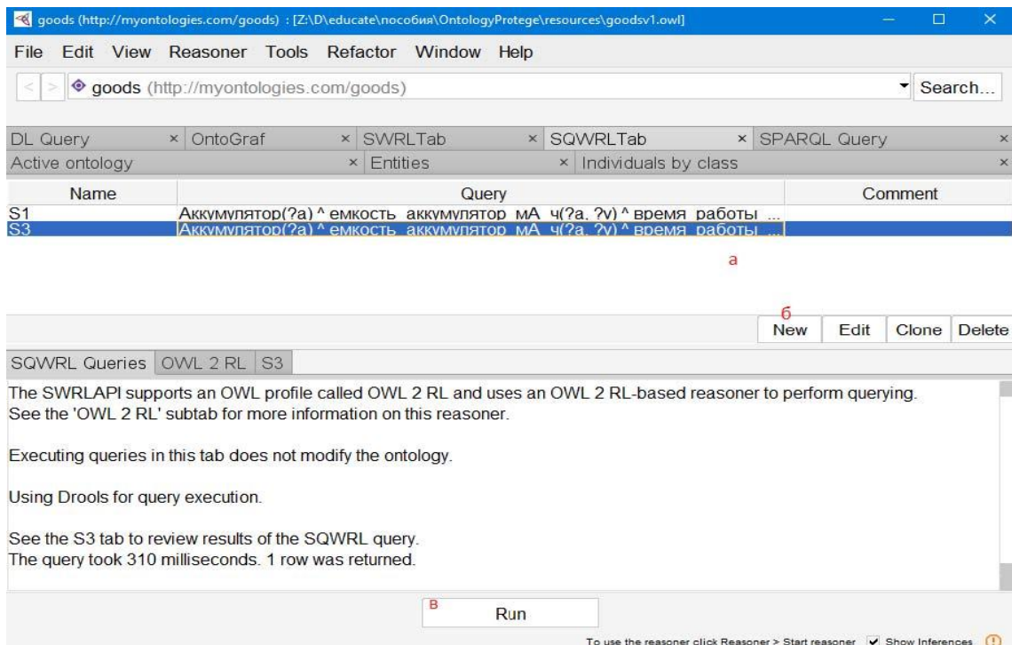
Рисунок 24 Вкладка SQWRL в системе Protégé (а – список созданных правил; б – кнопки создания нового правила и редактирования выделенного; в – кнопка запуска выбранного правила)
