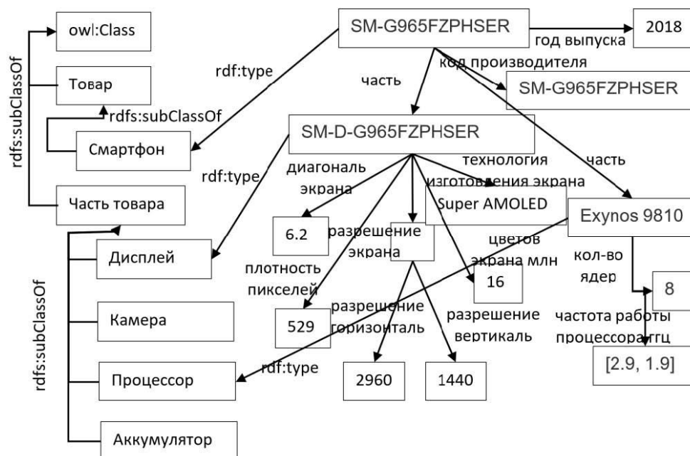
Рисунок 2 Фрагмент графа, описывающего классы, экземпляры и их отношения в рамках описания смартфонов
