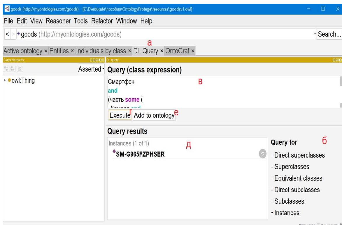
Рисунок 20 Вкладка «DLQuery» в системе Protégé (а – панель вкладок с активной вкладкой «DLQuery»; б – панель выбора типа запрашиваемых сущностей; в – поле ввода запроса; г – кнопка выполнения запроса; д – результаты запроса; е – кнопка добавления запроса в онтологию)
