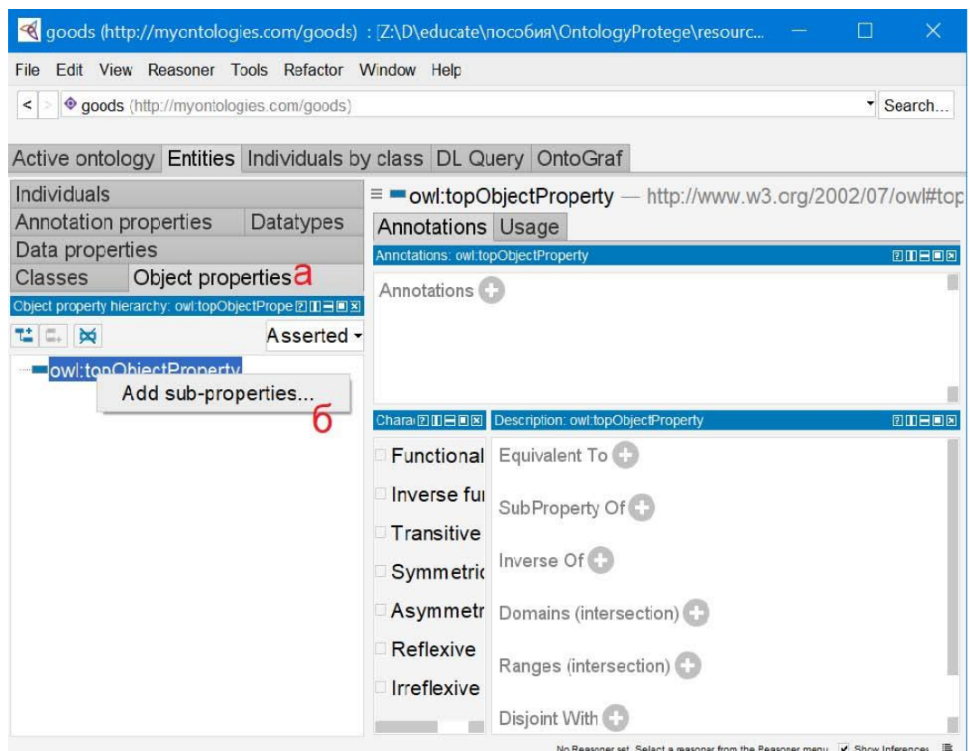
Рисунок 8 Добавление Object Properties, а – активная вкладка Object Properties, б – кнопка добавления иерархии отношений)
