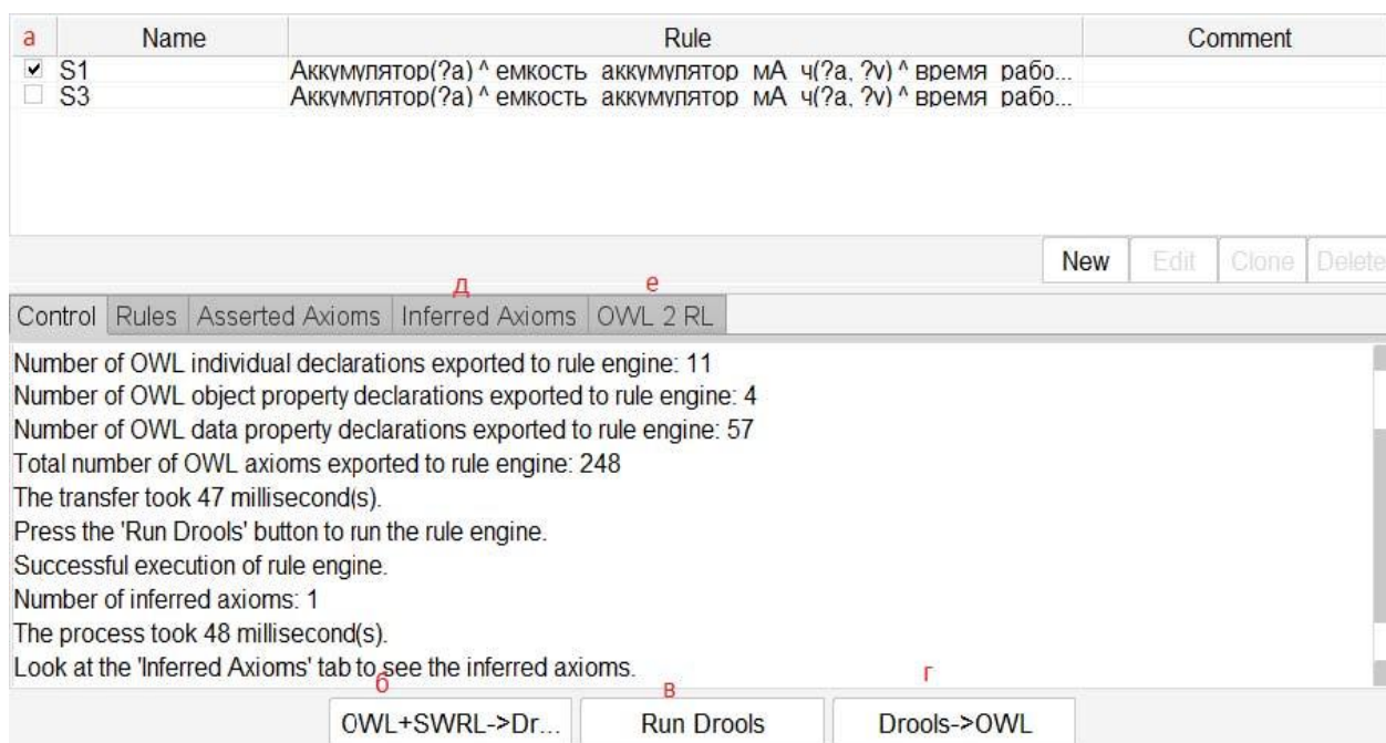
Рисунок 26 Вкладка SWRL в системе Protégé (а – активность правила; б – кнопка загрузки понятий/аксиом из онтологии и списка правил; в – запуск вывода на основе правил; г – внесение выведенных понятий в онтологию; д – список выведенных понятий; е – настройки вывода)
