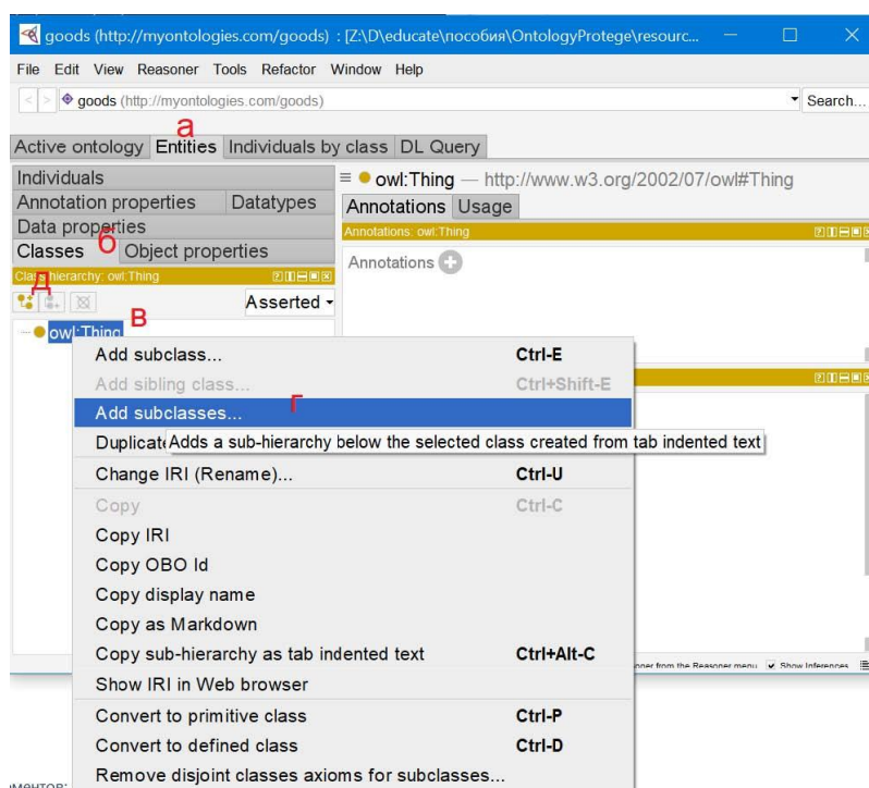
Рисунок 5 Вкладка «Entities» в системе Protégé (а – панель в вкладках с активной вкладкой «Entities»; б – панель вложенных вкладок вкладки «Entities» с активной вкладкой «Classes»; в – суперкласс owl:Thing; г, д – кнопки добавления иерархии подклассов/подкласса для выделенного класса)
