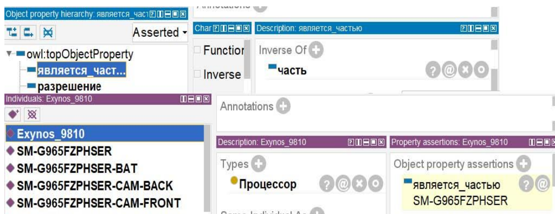
Рисунок 19 Демонстрация вывода в соответствии с описанием inverseOf
