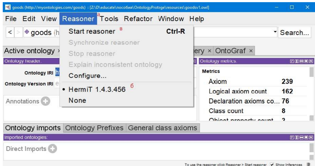
Рисунок 16 Запуск механизма вывода в системе Protégé (а – пункт меню с действиями вывода, б – выбранный механизм HermiT, в – кнопка запуска вывода).
