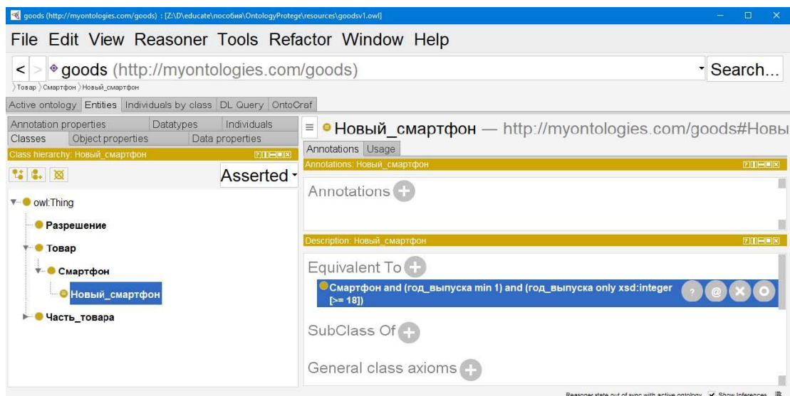
Рисунок 22 Пример заполнения поля «Equivalent To» в описании класса
