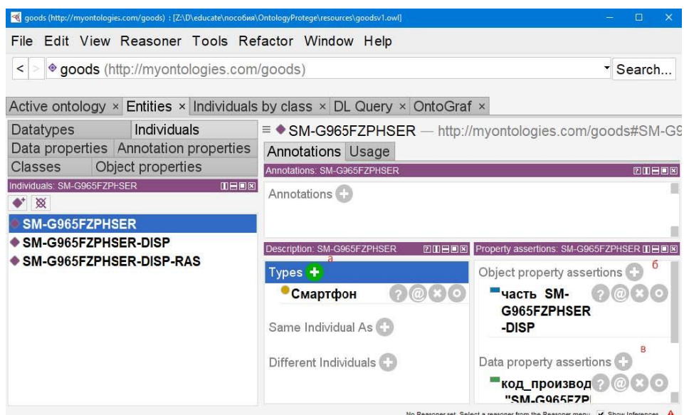
Рисунок 13 Окно описания экземпляра в системе Protégé (а – задание отношения rdf:type , б – задание отношений с использованием object property , в – задание отношений с использованием data property )
