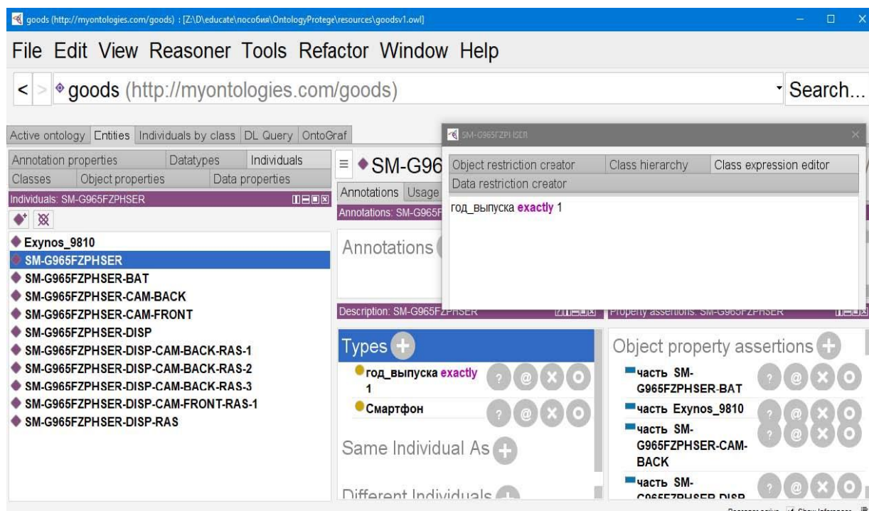
Рисунок 21 Использование вкладки «Class expression editor» для добавления информации о экземпляре
