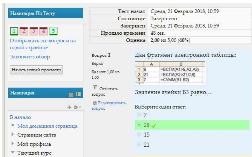
Рисунок 27. Результат тестирования
