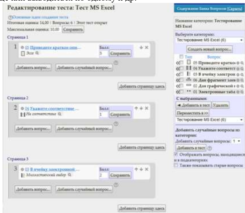
Рисунок 24. Созданный тест
