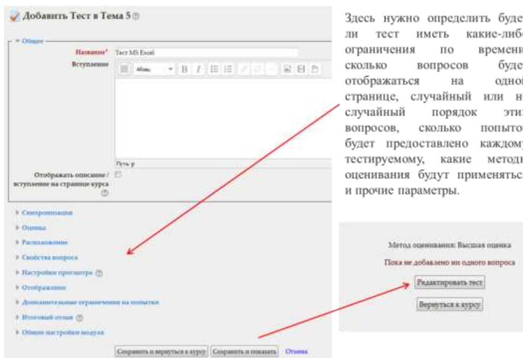
Рисунок 22. Настройка теста
