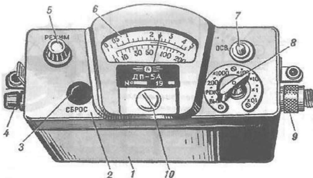
Рисунок 2.7 – Измерительный пульт рентгенометра дозиметра ДП-5 А: 1 — кожух; 2 — панель; 3 — кнопка сброса показаний микроамперметра; 4 —
