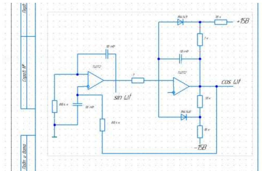
Рис. 11. Готовая схема
