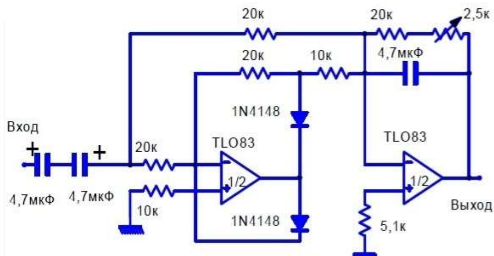
Выпрямитель двухполупериодный
