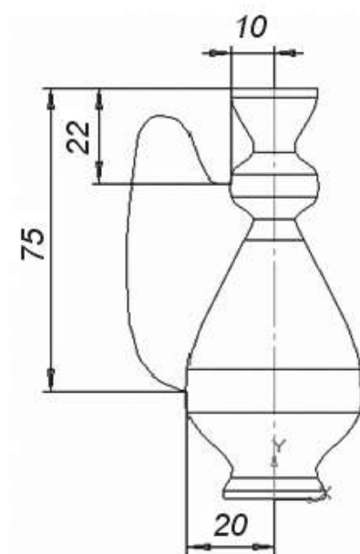
Рис. 8.16. Сечение объекта
