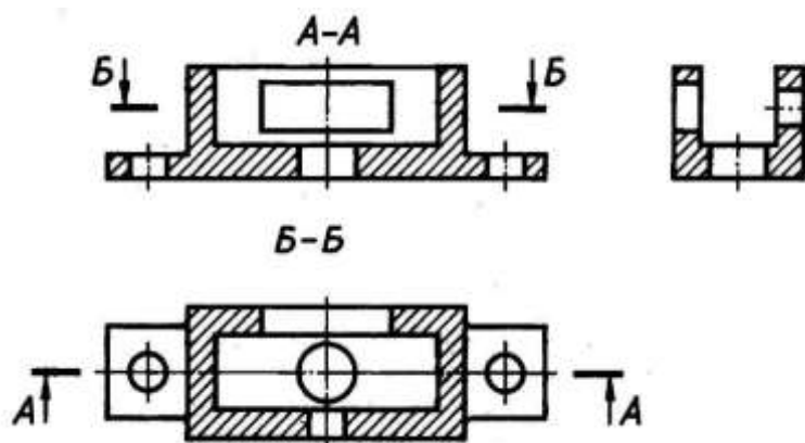
Рис. 6.7. Обозначение разрезов
