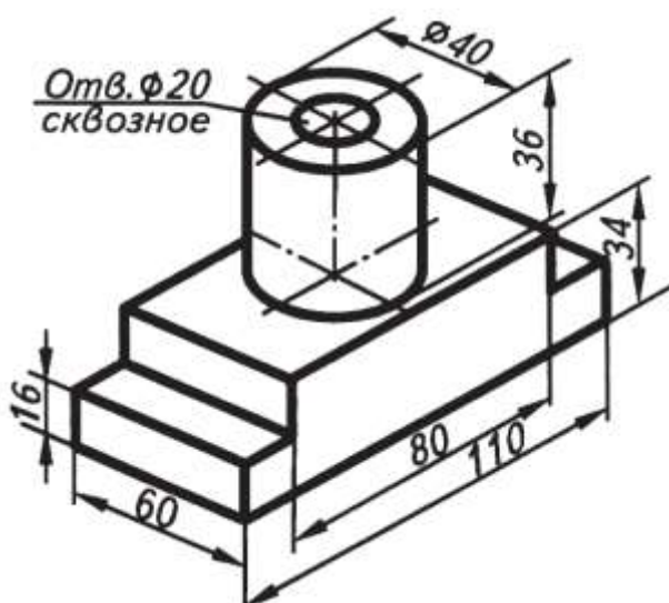
Рис. 7.3. Построение детали
