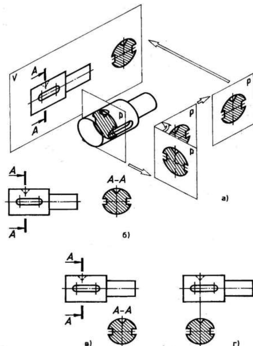
Рис. 6.2. Сечения:
