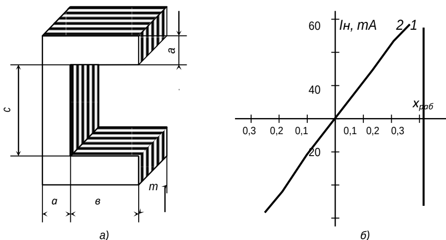
Рис1. Конструкция (а) и статические характеристики (б)
