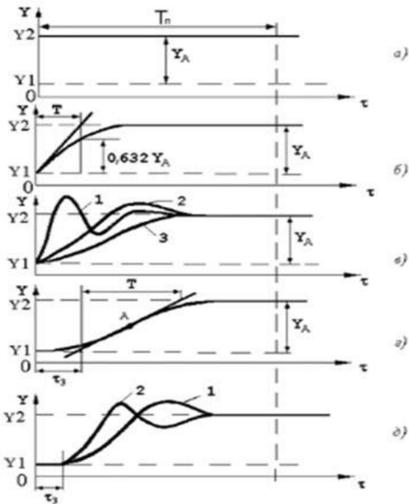
Рисунок 1. Переходные процессы.
