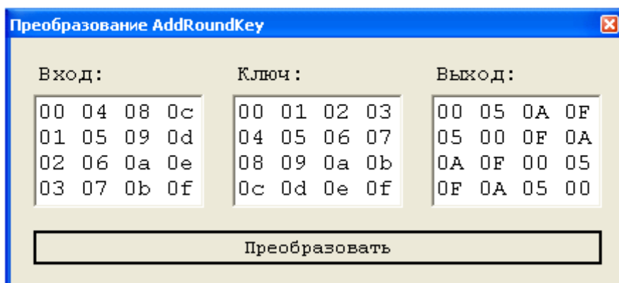
Рисунок 5. Окна преобразований MixColumn и AddRoundKey
