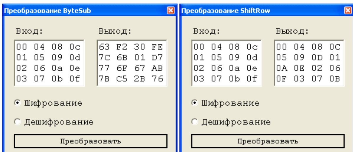
Рисунок 4. Окна преобразований ByteSub и ShiftRow
