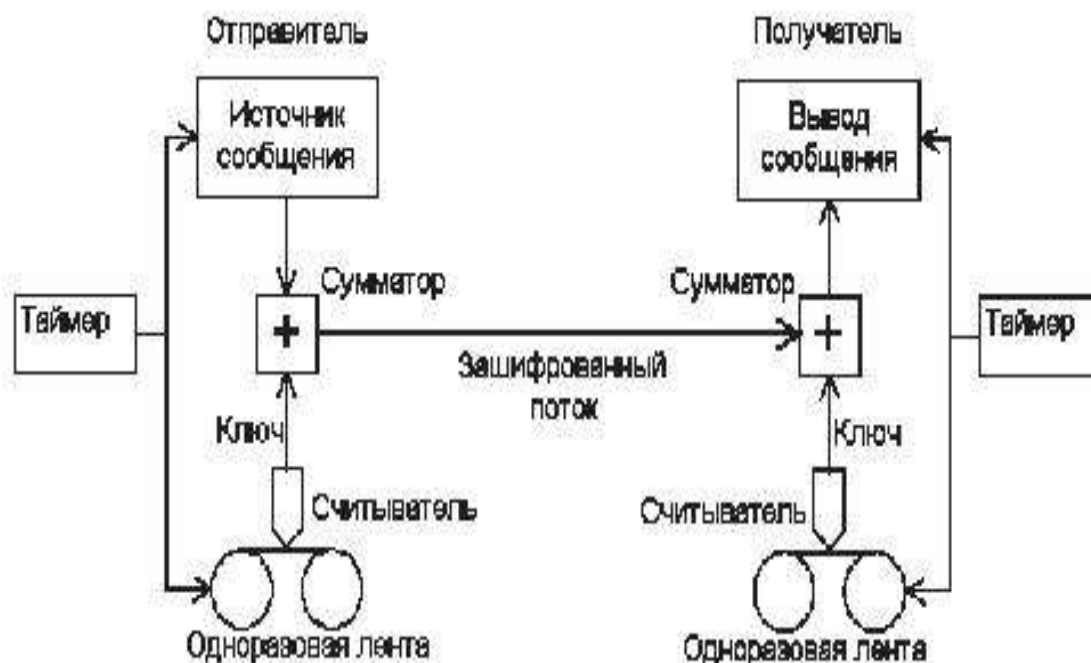
Рис. 1.1. Шифрование методом Вернама
