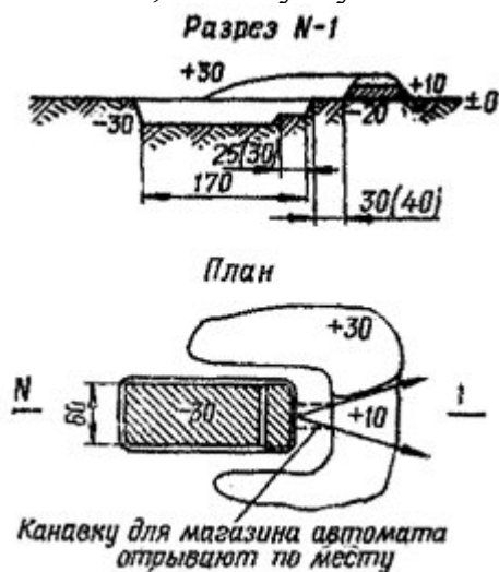
Одиночный окоп для стрельбы из автомата лежа
