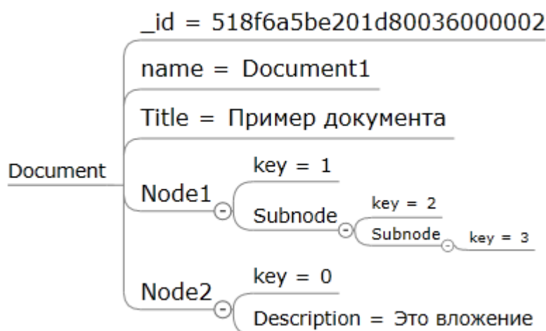
Рисунок 1 – Пример документа в NoSQL БД.
