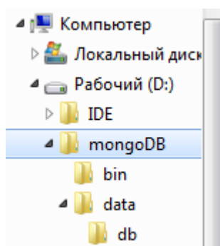
Рисунок 5 – Иерархия папок в MongoDB
