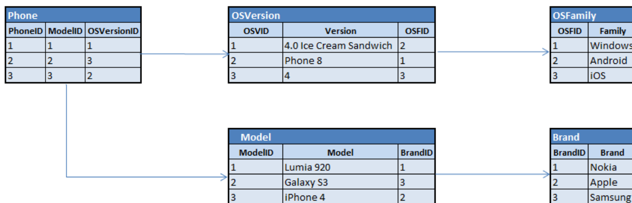
Рисунок 2 – Схема базы данных «телефон».
