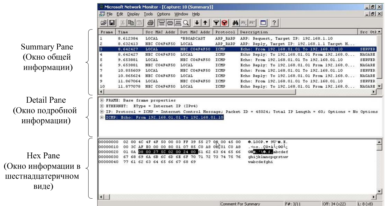
Рис. 6. Элементы окна Summary
