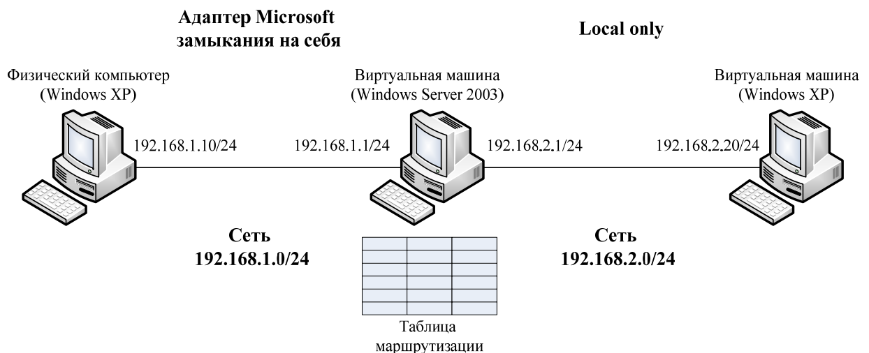
Рис. 4. Схема сети с маршрутизатором
