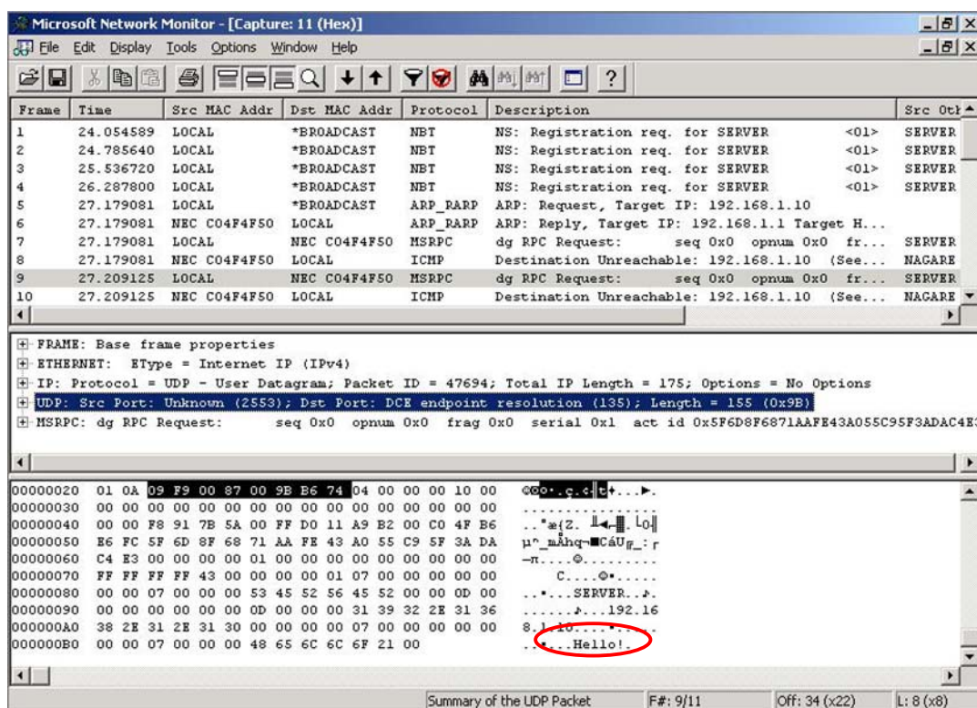
Рис. 7. Перехват текстового сообщения
