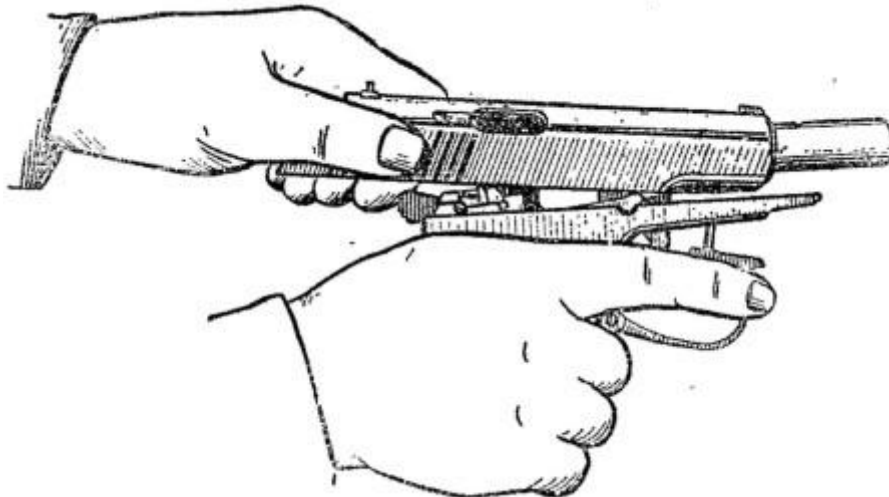
Рис. 5. Отделение затвора от рамки
