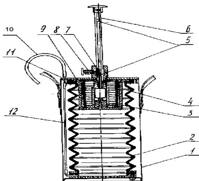
Рис. 12. Газоанализатор УГ-2
