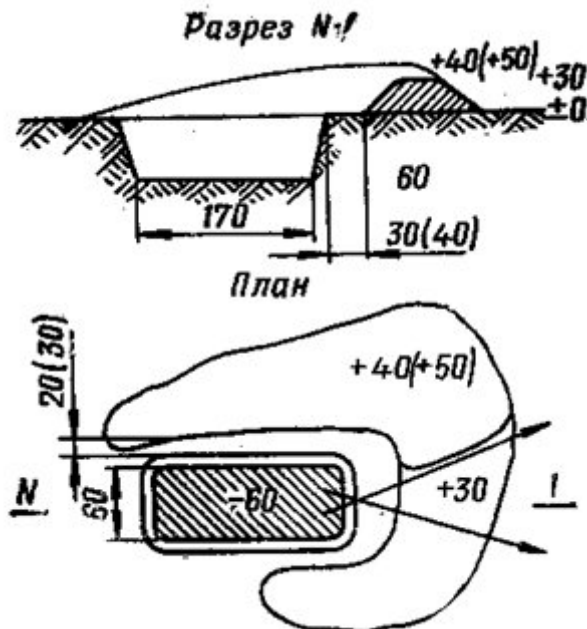
Одиночный окоп для стрельбы из автомата с колена
