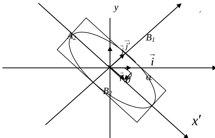
Рис.1. Эллипс, заданный уравнением.
