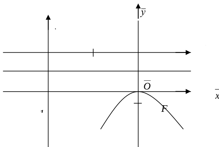
Рис.2.Парабола, заданная уравнением
