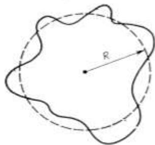
Рисунок 1 – Расширяющаяся зона нарушения режима в неоднородном пласте
