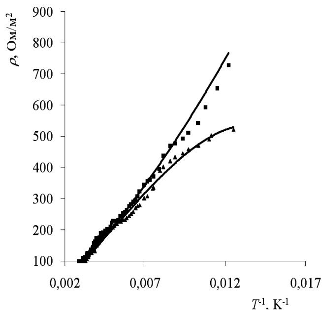
Рисунок 1 – Температурные зависимости удельного сопротивления плёнок a -SiC:H
