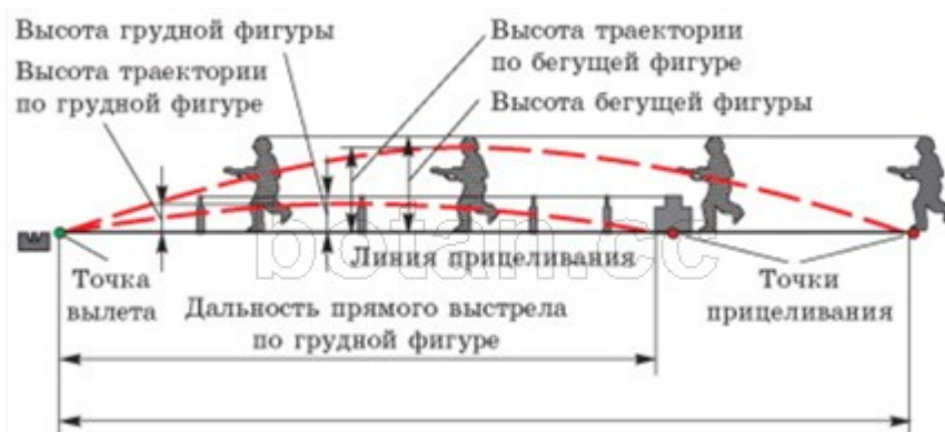
Рис. 51. Прямой выстрел
