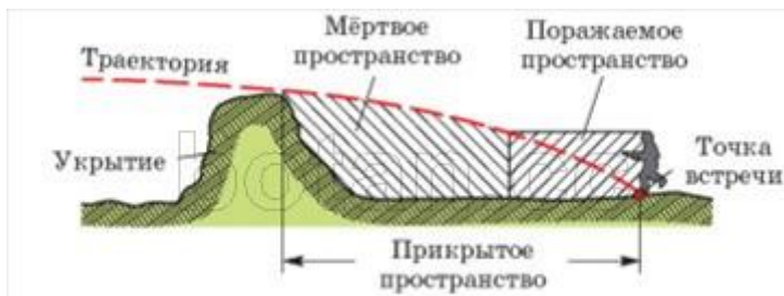
Рис. 52. Прикрытое, поражаемое и мёртвое пространство
