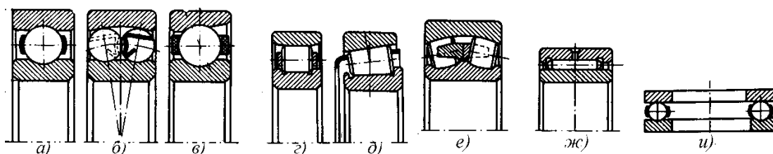
Рисунок 5.2 – Типы подшипников качения
