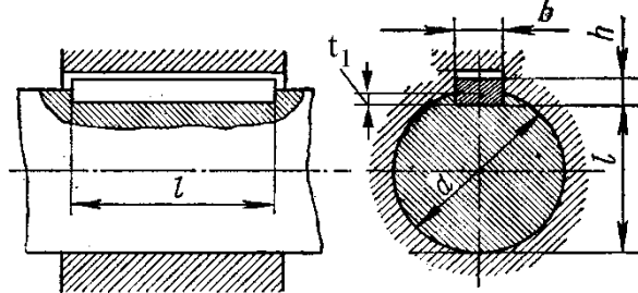
Рисунок 12 – Расчетная схема
