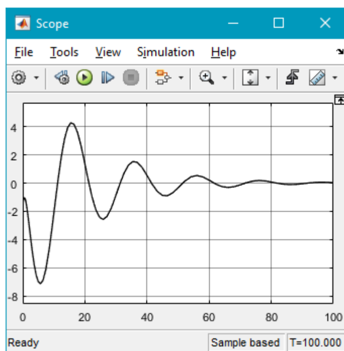
Рисунок 11.2 – Движение физического маятника
