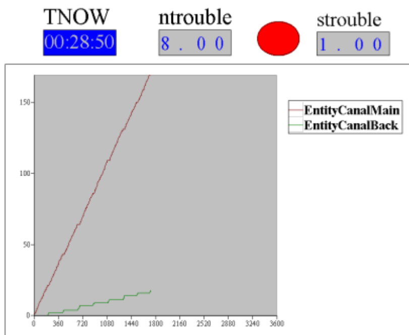
Рисунок 13.19 – Результаты анимации
