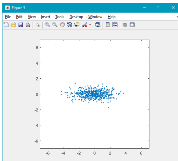
Рисунок 3.19 – Сгенерированное множество точек для случая
