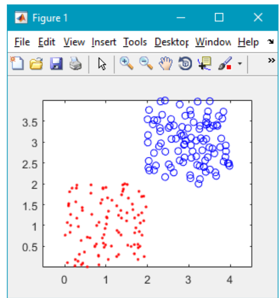
Рисунок 4.2 – Два класса для X_2
