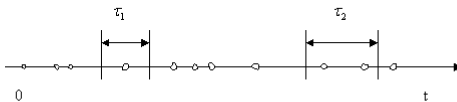
Рисунок 9.2. – Изображение потока событий на оси времени
