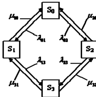
Рисунок 9.3. – Размеченный граф состояний системы
