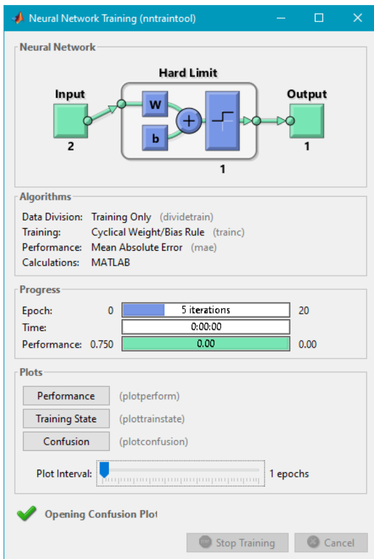
Рисунок 3.10 – Нейронная сеть, реализующая конъюнкцию – а ; настройка весов обучения – б ; результат работы сети – с
