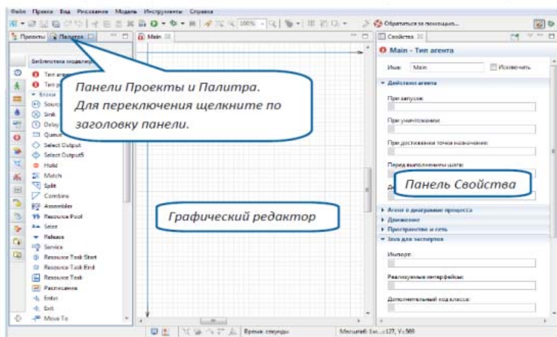
Рисунок 14.1 – Интерфейс среды имитационного моделирования AnyLogic
