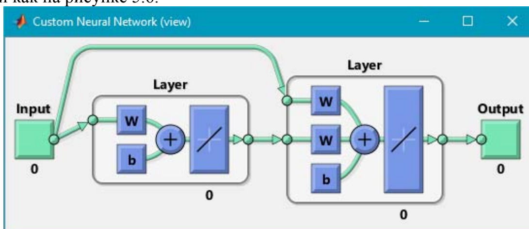
Рисунок 5.6 – Добавилась связь входа со вторым слоем
