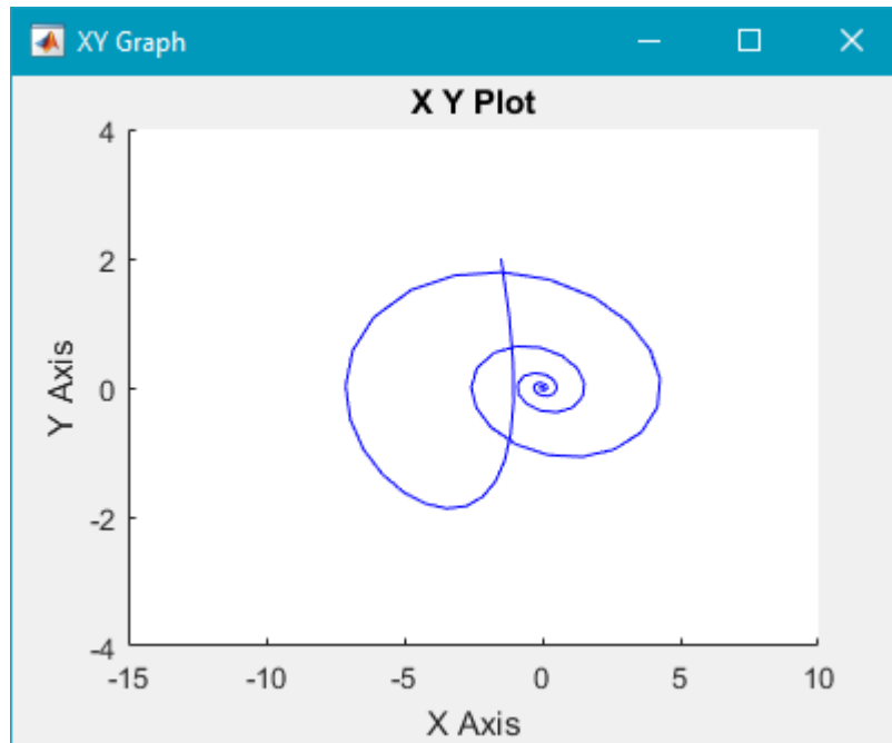
Рисунок 11.3 – Фазовый портрет физического маятника
