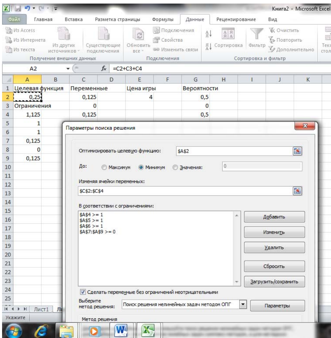
Рисунок 8.3 – Рабочий лист с результатами решения задачи для первого игрока и заполненными полями окна диалога «Параметры поиска решения»
