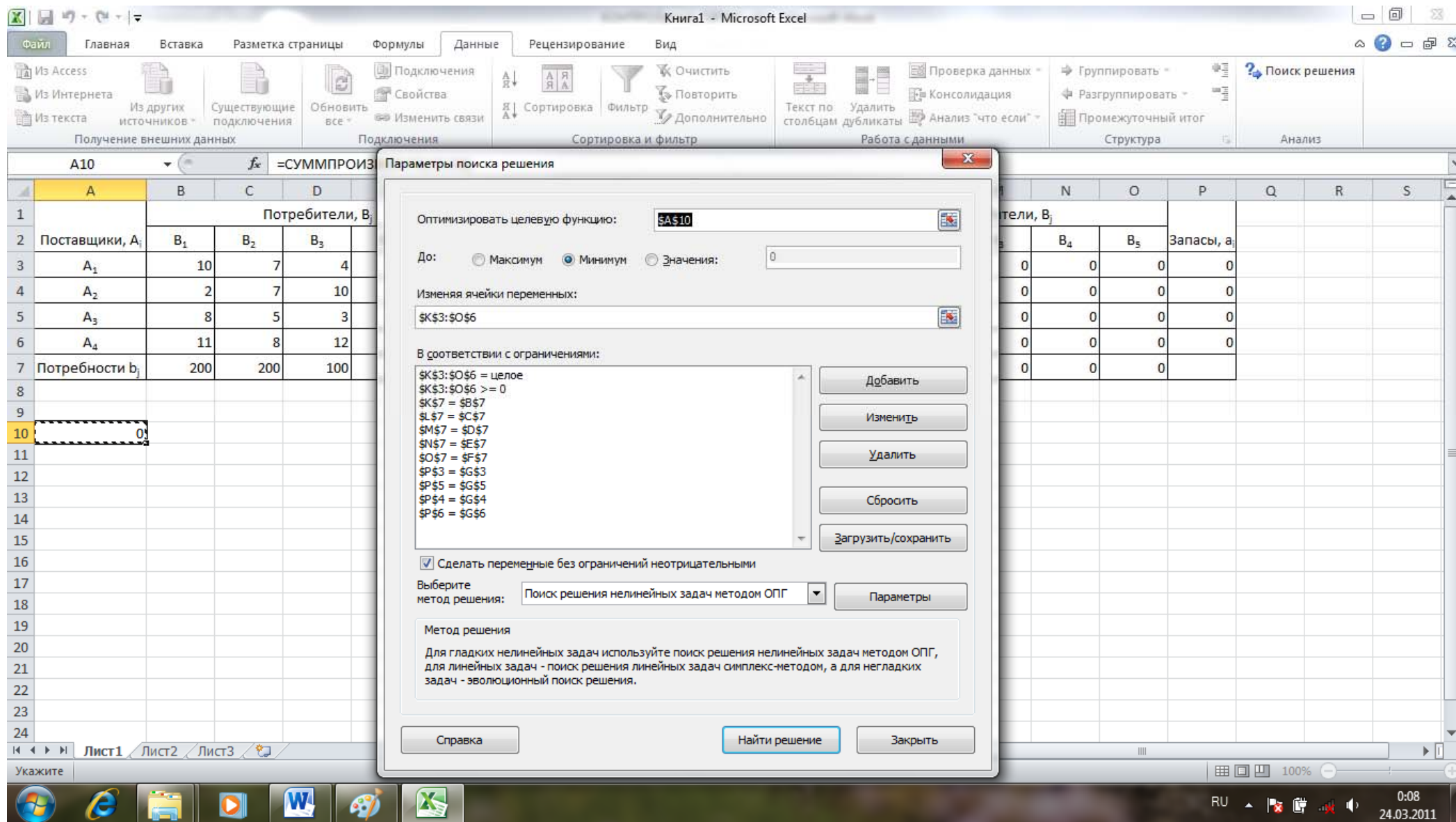
Рисунок 7.5 – Рабочий лист с введенными данными и окно диалога «Поиск решений»
