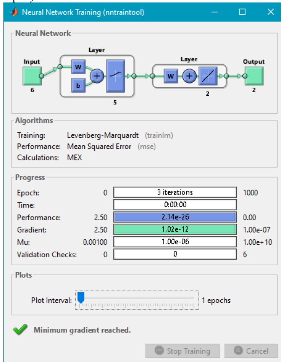
Рисунок 5.10 – Обучение сети
