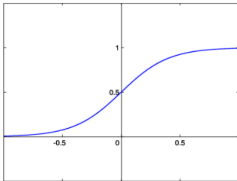
Рисунок 3.1 – График
