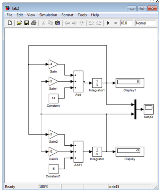
Рисунок 2.5 – Структурная схема модели системы дифференциальных уравнений 2. 6
