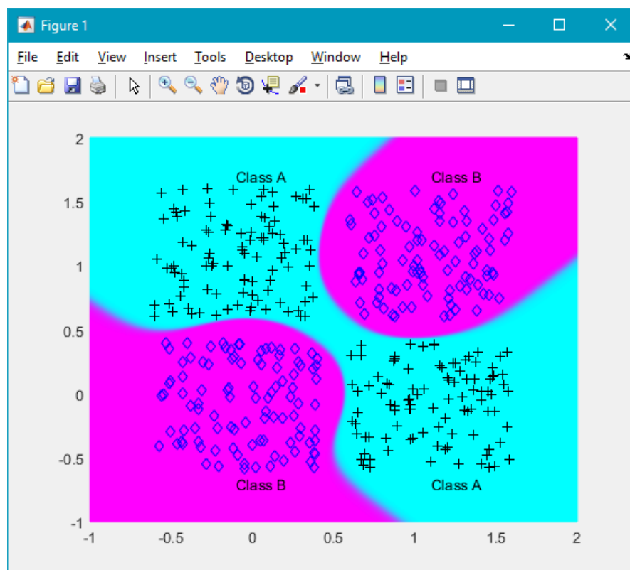
Рисунок 5. 31 – Граница решений для сети с пятью скрытыми нейронами Сеть со структурой 2-3-1 даст ошибку, показанную на рисунке 5.32.
