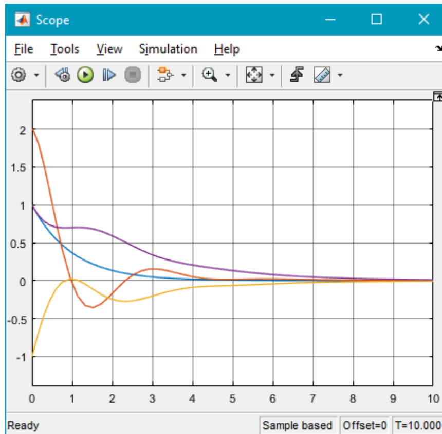
Рисунок 11.6 – Переходный процесс системы
