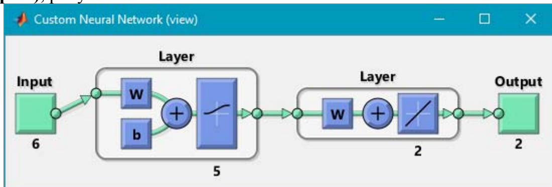
Рисунок 5.9 – Окончательно получаем общую структуру сети, где размер входа – 6, а выхода – 2
