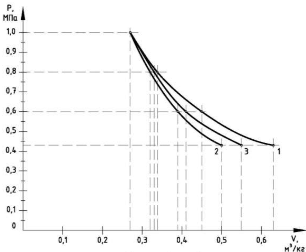
Рисунок 1. P-v диаграмма
