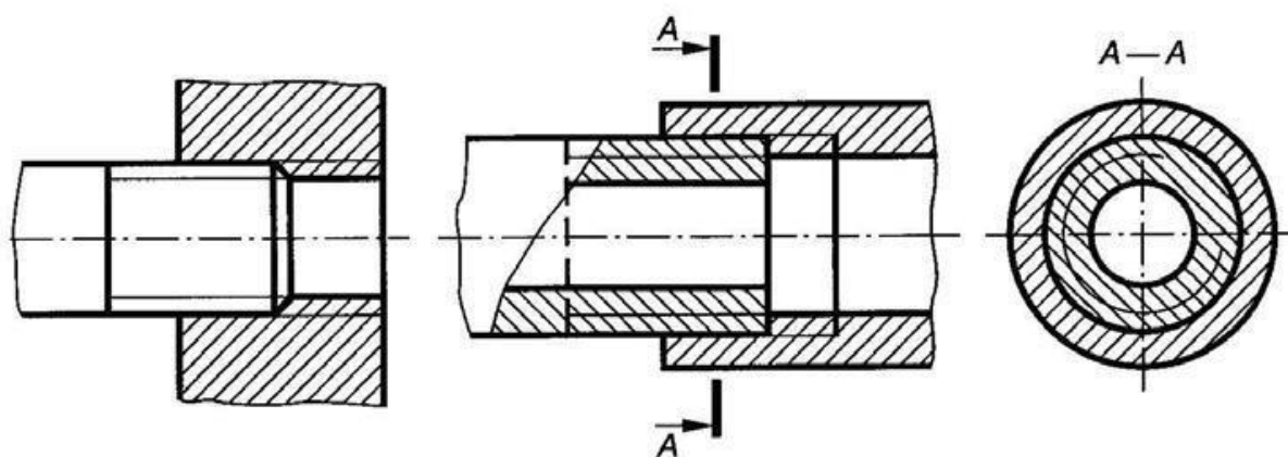
Рисунок 29.4 – Соединение резьбовое
