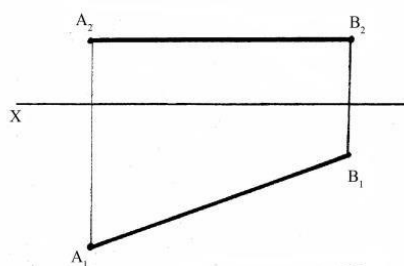
Рисунок 6.3- Горизонталь
