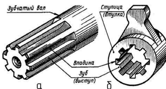
Рисунок 30.3 – Детали со шлицами
