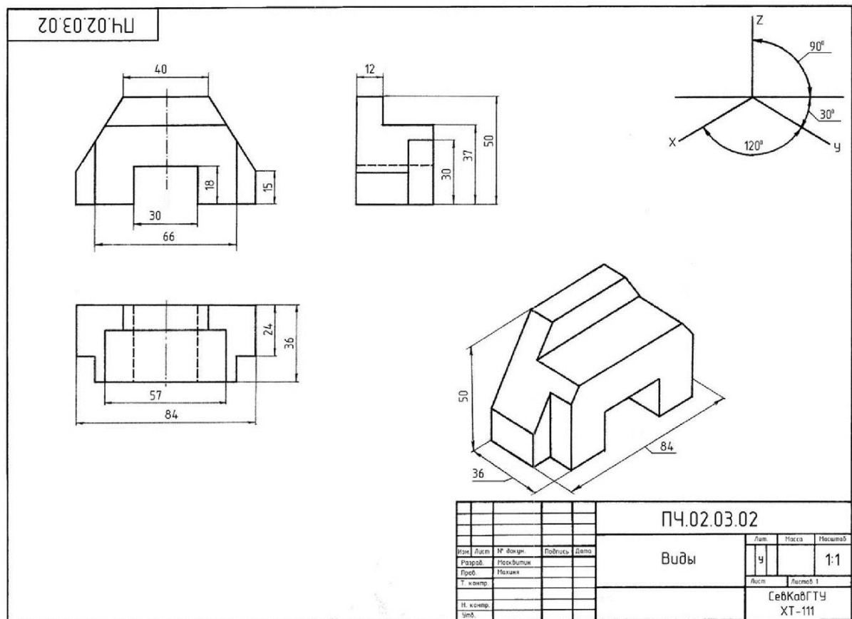
Рисунок 22.5 – Пример выполнения задания 22.1
