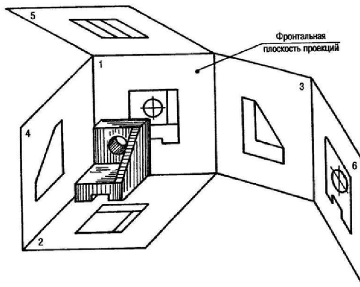
Рисунок 22.1 – Образование видов
