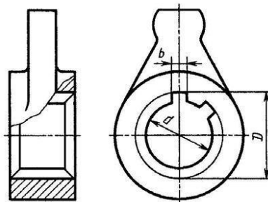
Рисунок 30.6 – Шлицевая ступица
