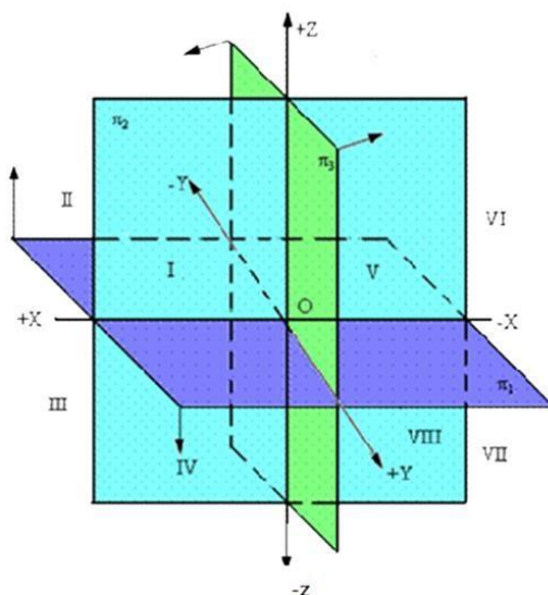
Рисунок 4.1 – Октанты пространства
