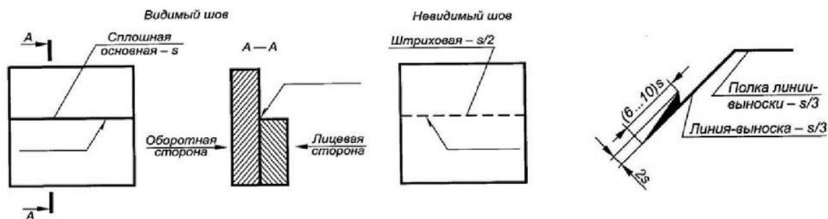
Рисунок 31.2 – Изображение швов
