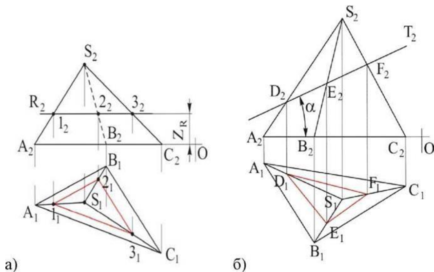
Рисунок 14.1 — Сечение пирамиды плоскостями частного положения
