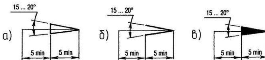
Рисунок 22.3 – Стрелки
