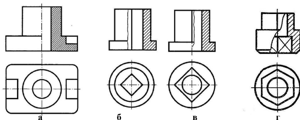
Рисунок 23.8 – Совмещение вида с разрезом
