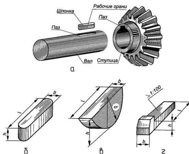
Рисунок 30.1 – Виды шпонок
