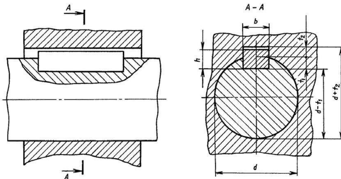
Рисунок 30.2 – Соединение шпоночное
