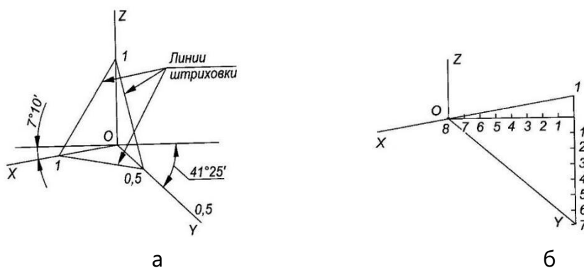
Рисунок 28.1 – Оси координат в диметрии
