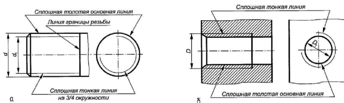
Рисунок 29.3 – Изображение резьбы
