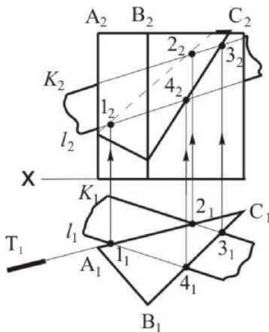
Рисунок 14.2 — Прямая призма (способ граней)
