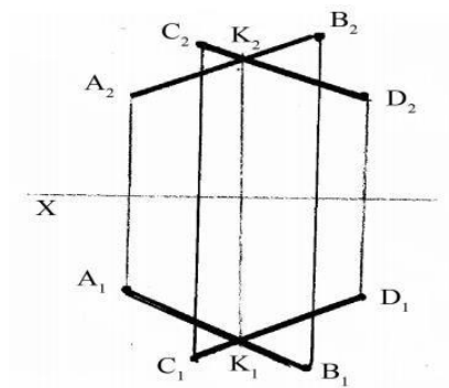
Рисунок 7.2 – Эпюр пересекающихся прямых
