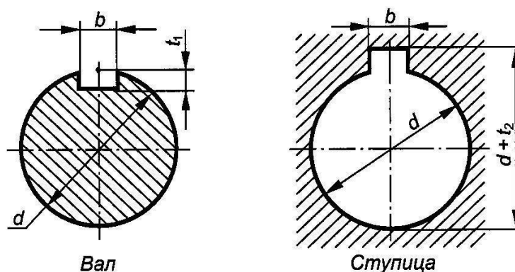
Рисунок 26.5–Размеры шпоночного паза
