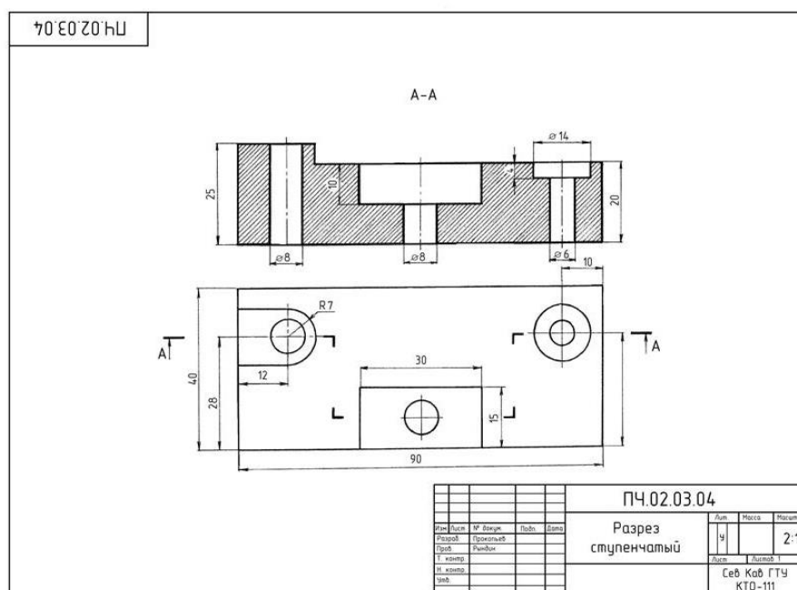
Рисунок 24.2 – Пример выполнения задания 24.1
