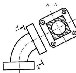
Рисунок 23.5 – Наклонный разрез
