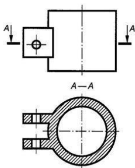
Рисунок 23.2 – Горизонтальный разрез
