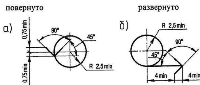
Рисунок 22.4 – Знаки
