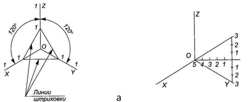
Рисунок 27.2 – Оси координат в изометрии
