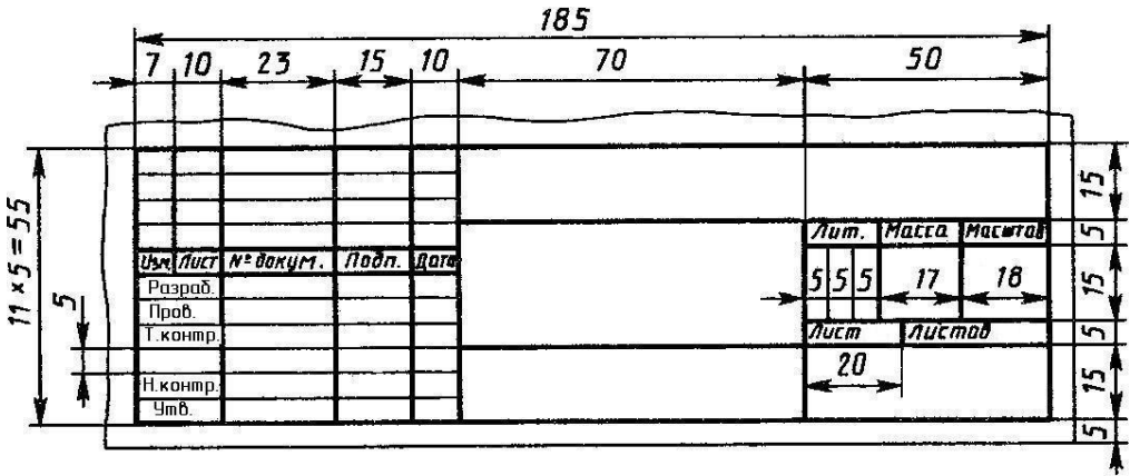
Рисунок 2.2 – Основная надпись
