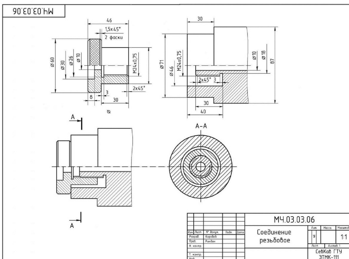
Рисунок 29.6 – Пример выполнения задания 29.1
