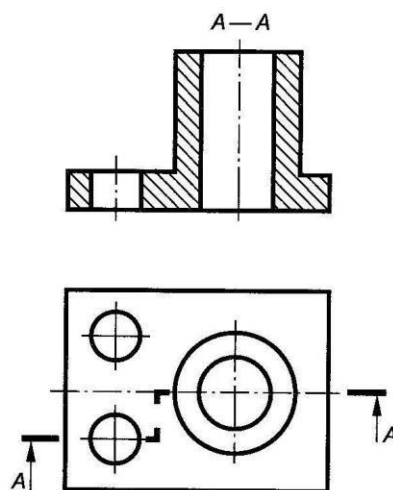
Рисунок 24.1 – Разрез ступенчатый
