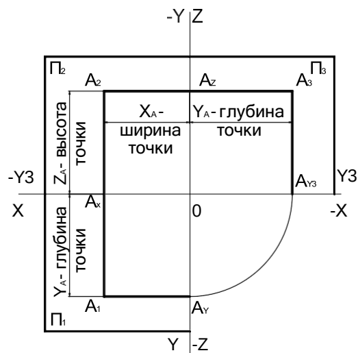
Рисунок 4.2 – Эпюр точки А с указанием координат
