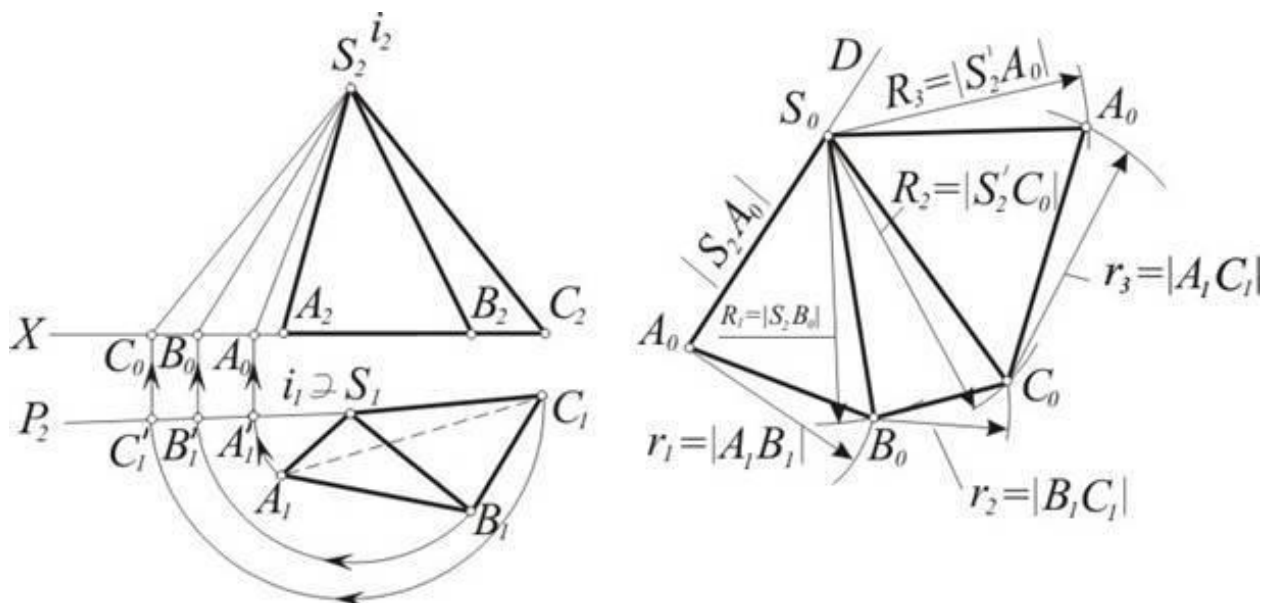
Рисунок 18.1 – Развертка пирамиды способом триангуляции
