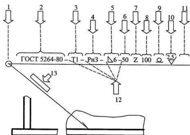
Рисунок 31.4 – Структура обозначения шва: 1 – шов по замкнутому контуру; 2 – номер стандарта; 3 – буквенно-цифровое обозначение шва: Т1 – тавровый, односторонний; 4 – способ сварки: РнЗ – ручная электродуговая неплавящимся электродом в защитных газах; 5 – катет шва и его размер: К=6 мм; 6...8 – шов прерывистый шахматный длиной 50 мм и шагом 100 мм; 9 – усиление шва снять; 10 – шероховатость поверхности; 11 – место для знака, что шов выполнен по незамкнутой линии; 12 – дефис; 13 – указание о контроле шва
