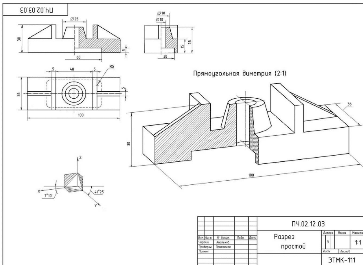
Рисунок 23.9 – Пример выполнения задания 23.1
