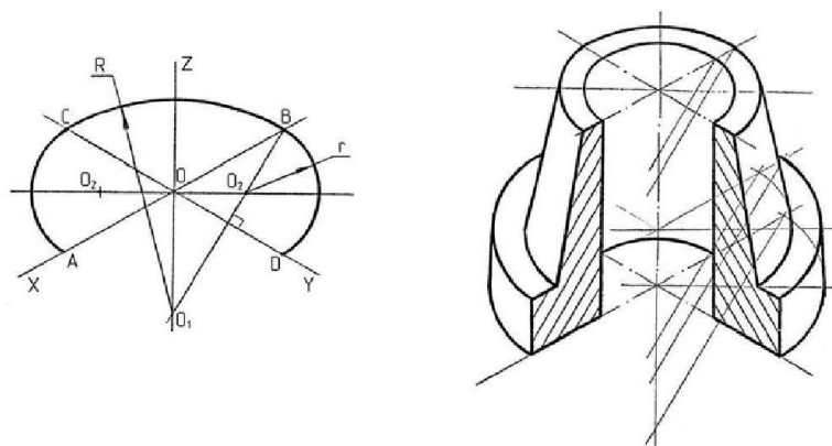
Рисунок 27.4 – Овал в изометрии и деталь с четвертью выреза
