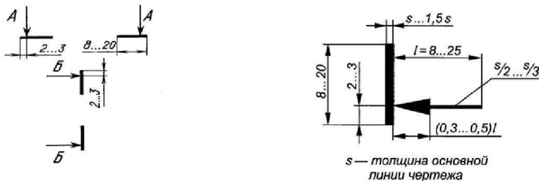
Рисунок 23.6 – Линия сечения
