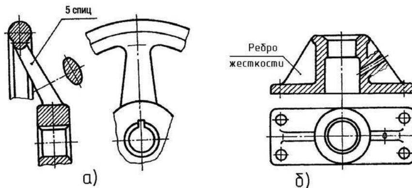
Рисунок 23.7 – Условности разрезов
