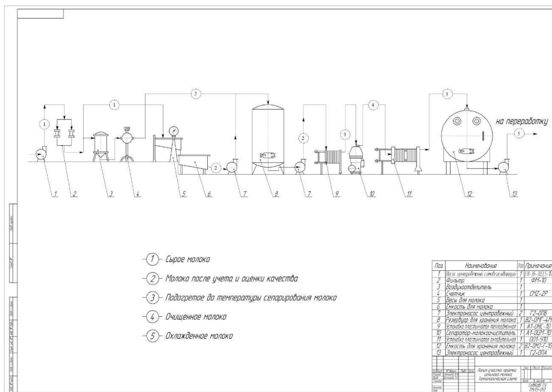
Рисунок 34.2 – Пример выполнения задания 34.1
