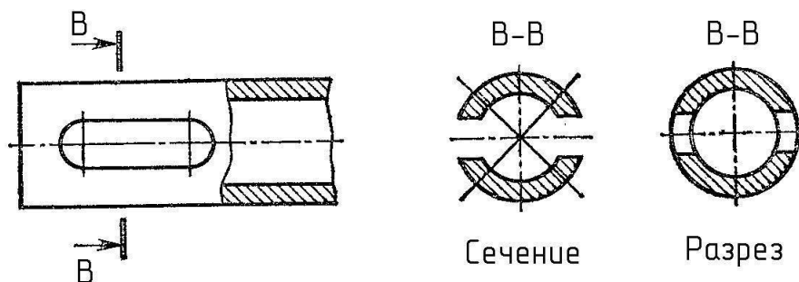
Рисунок 26.4 – Сечение не круглого отверстия
