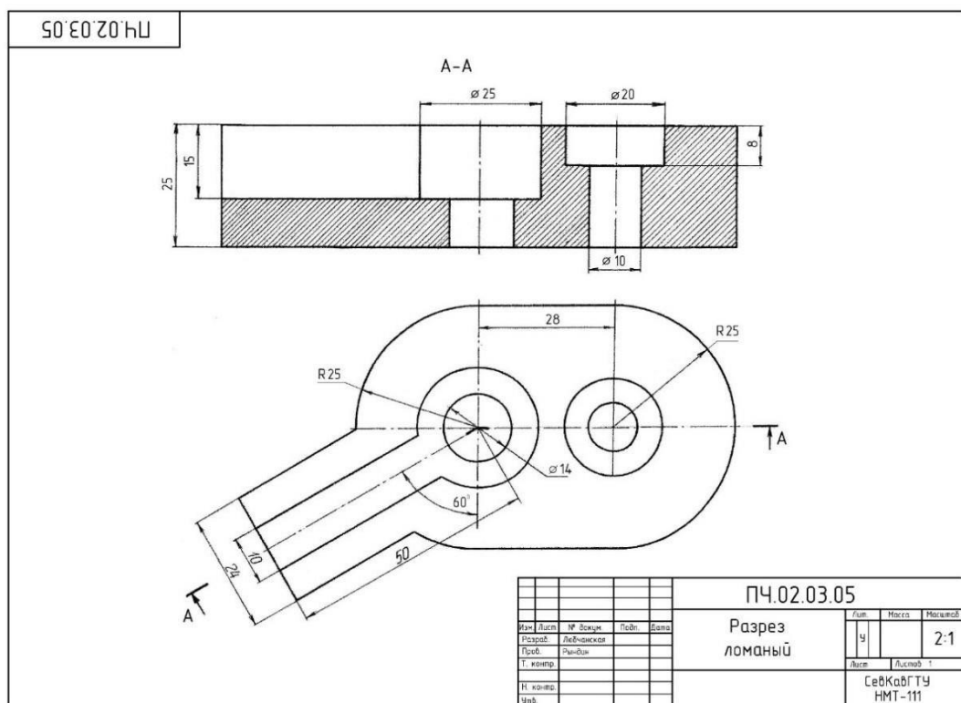
Рисунок 25.2 – Пример выполнения задания 25.1
