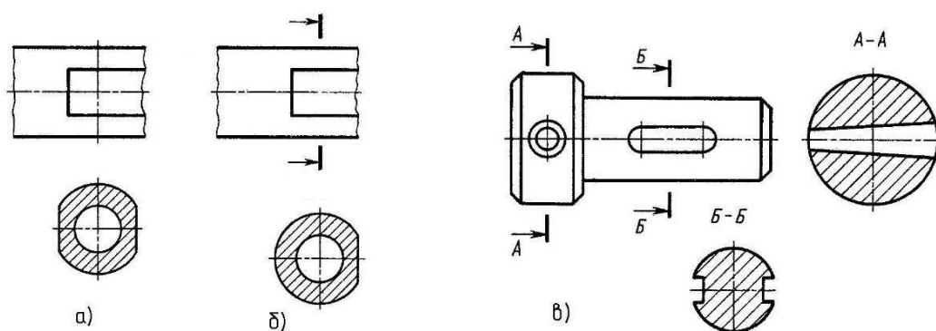
Рисунок 26.3 – Варианты расположения вынесенного сечения
