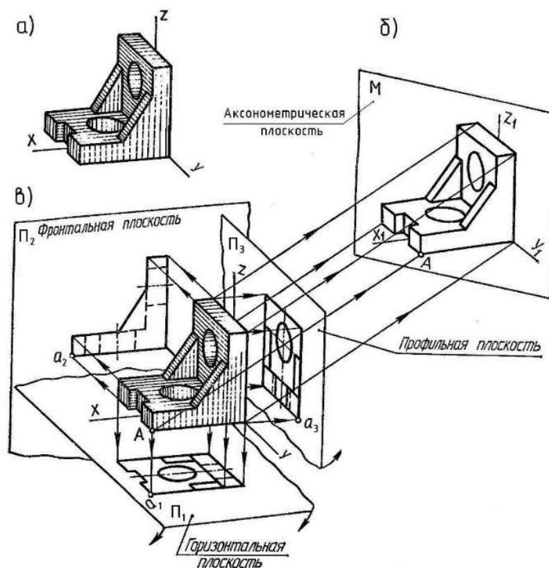
Рисунок 27.1 – Образование аксонOMETрии
