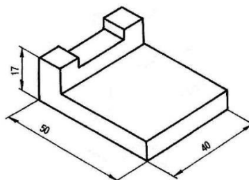
Рисунок 27.3 – Изометрия детали с габаритными размерами
