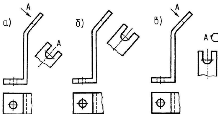
Рисунок 22.2 – Дополнительные виды
