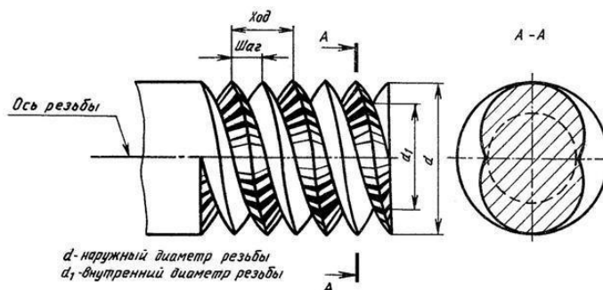
Рисунок 29.1 – Резьба цилиндрическая двухзаходная
