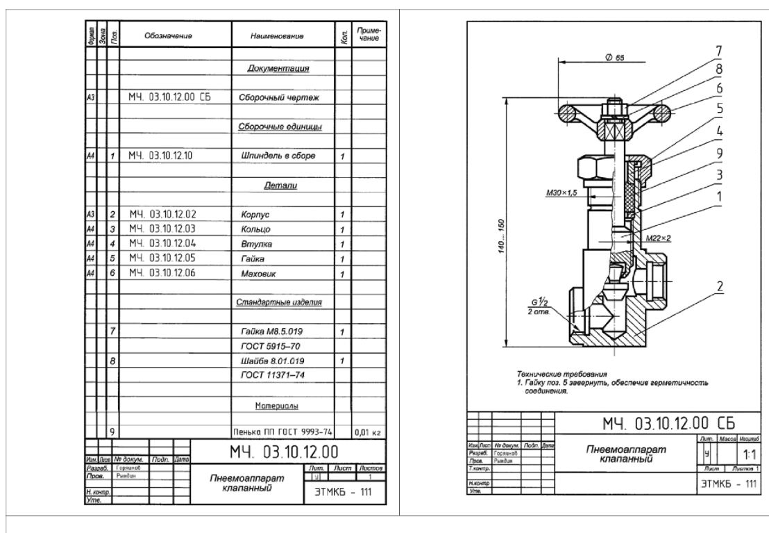
Рисунок 32.2 – Пример выполнения задания 32.1
