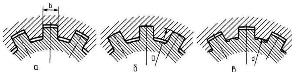
Рисунок 30.4 – Способы центрирования ступицы и вала
