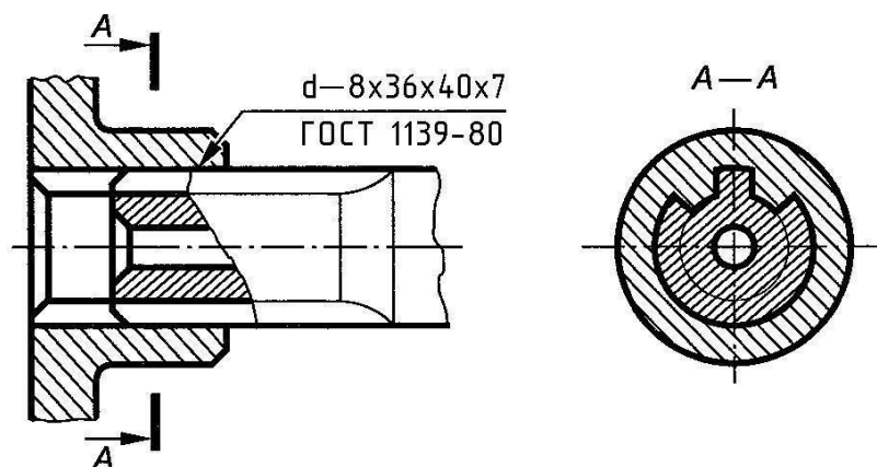
Рисунок 30.7 – Соединение шлицевое
