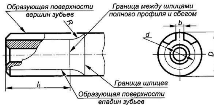
Рисунок 30.5 – Шлицевой вал
