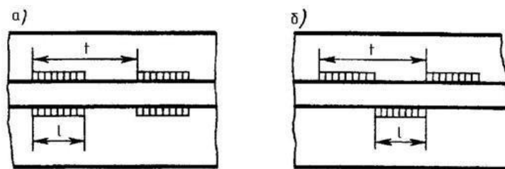
Рисунок 31.1– Типы сварных швов
