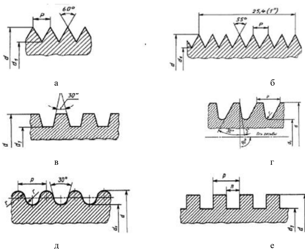
Рисунок 29.2 – Типы резьб
