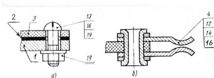
Рисунок 32.1 – Крепежная группа
