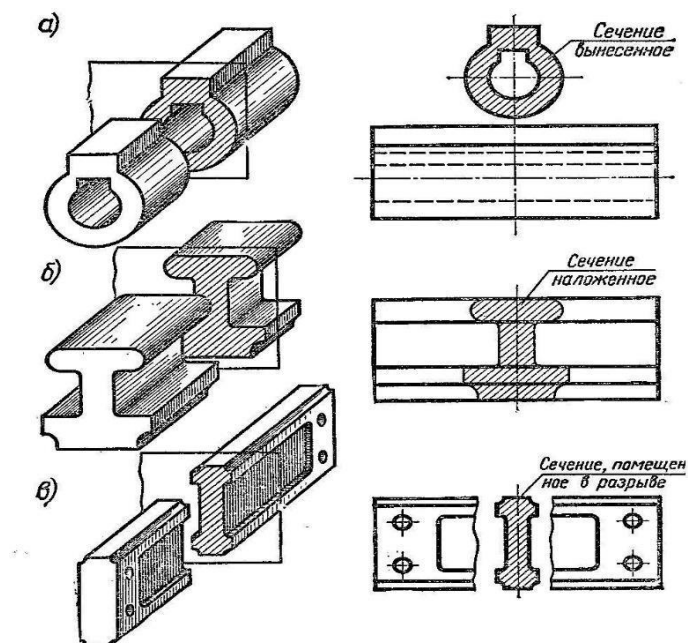
Рисунок 26.1 – Классификация сечений
