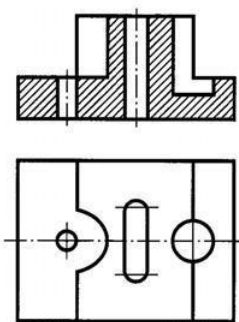
Рисунок 23.3 – Фронтальный разрез
