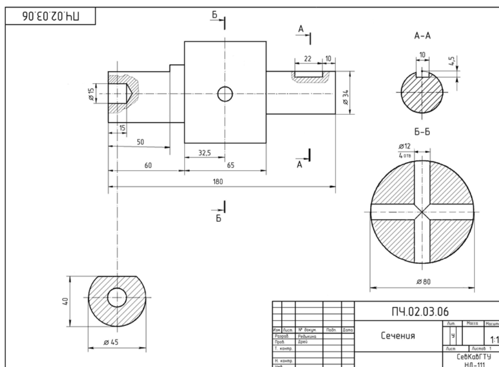
Рисунок 26.6 – Пример выполнения задания 26.1
