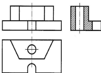
Рисунок 23.4 – Профильный разрез
