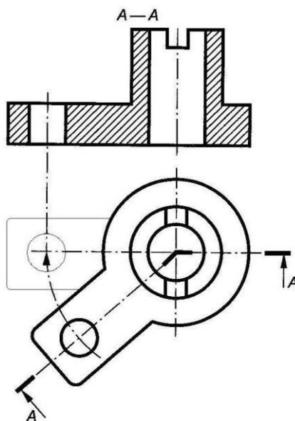
Рисунок 25.1 – Разрез ломаный
