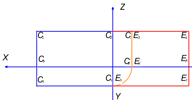
Рисунок 5.2 –Эюр симметричных точек
