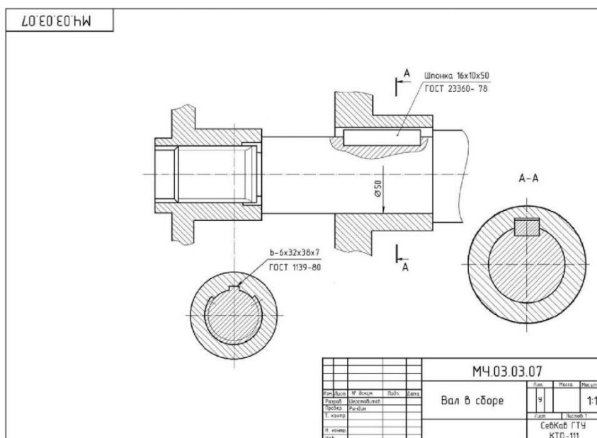
Рисунок 30.8 – Пример выполнения задания 30.1
