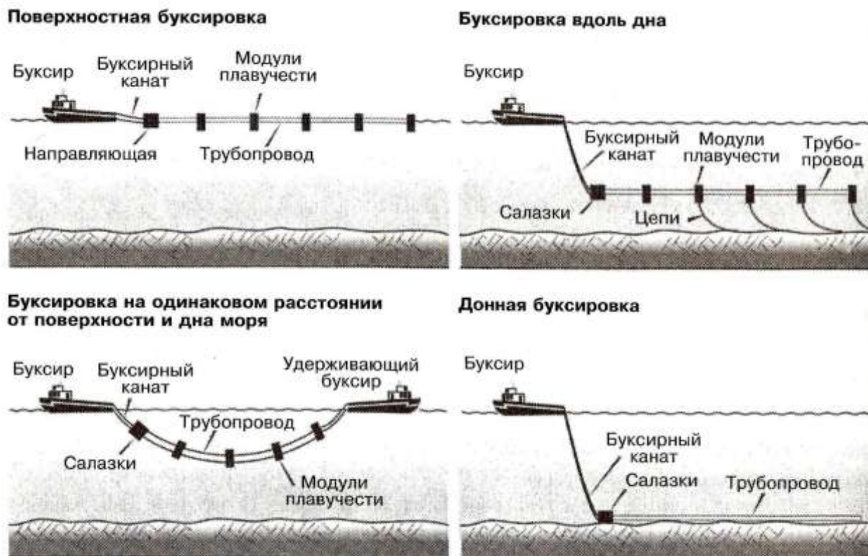
Рисунок 8 - Технологии буксировки и монтажа трубопровода
