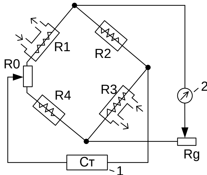
1 – источник стабилизированного напряжения; 2 – вторичный прибор; R_1 и R_3 – рабочие терморезисторы; R_2 и R_4 – сравнительные терморезисторы; R_0 и R_g – потенциометры; вход и выход анализируемой газовой смеси показаны стрелками.
