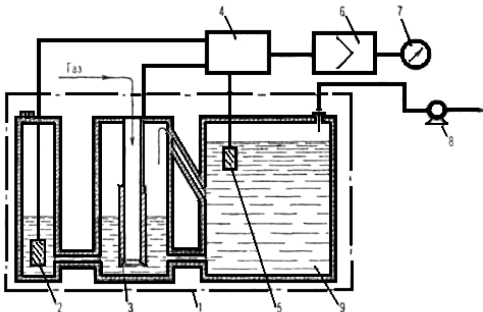
1 – электрохимическая ячейка; 2 – вспомогательный электрод; 3 – измерительный электрод; 4 – потенциостат; 5 – электрод сравнения; 6 – усилитель; 7 – измерительный прибор; 8 – побудитель расхода газа; 9 – камера с запасным электролитом.
