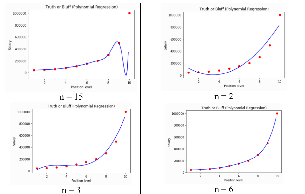
Рисунок 8.2 – Анализ модели полиномиальной регрессии
