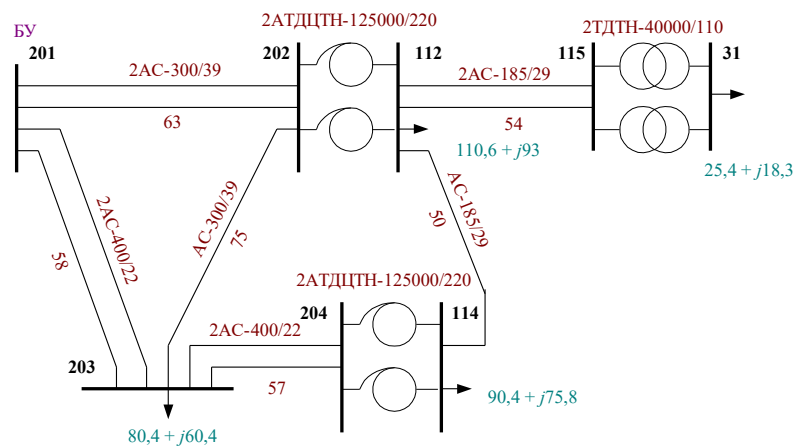
Рис.11.1. Схема существующей сети 220/110/35 кВ; длины линий в километрах, мощности нагрузок в мегавольт-амперах
