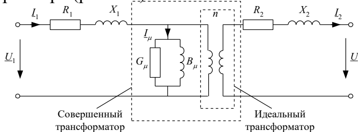
Рис. 3.1. Полная Т-образная схема замещения трансформатора
