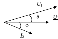
Рис. 3.5. Векторная диаграмма 2
