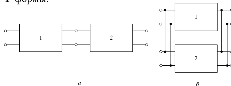
Рис. 6.1. Каскадное, (а) и параллельное, (б) соединения четырехполюсников
