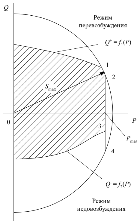
Рис. 7.1. Графическая модель располагаемой мощности гидрогенератора
