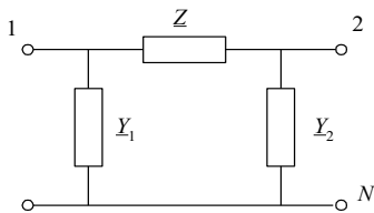
Рис. 3.3. П-образная схема замещения
