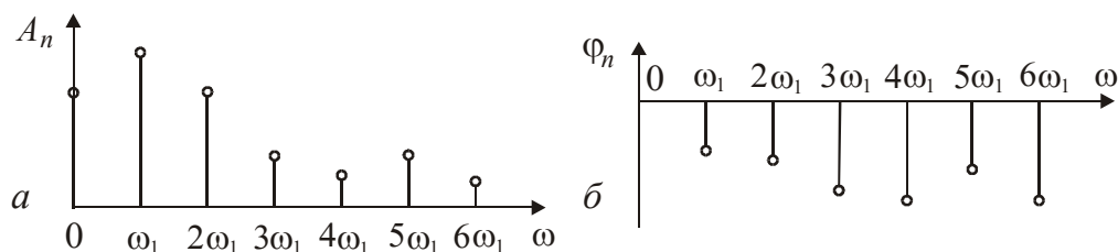
Рис. 1.1. Амплитудная и фазовая спектральные диаграммы
