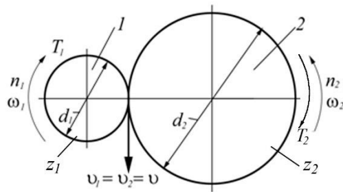
Рисунок 1 – Кинематика зубчатой механической передачи
