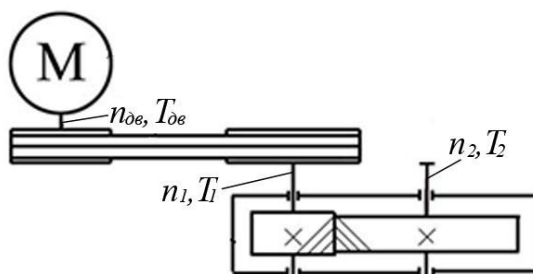
Рисунок 4 – Схема приводной станции
