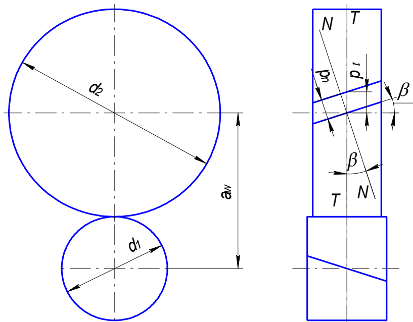
Рис. 3.2 – Косозубая передача
