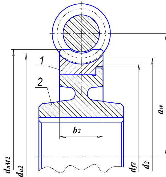
Рис. 5.2 – Червячное зацепление: 1 – венец червячного колеса; 2 – основание колеса
