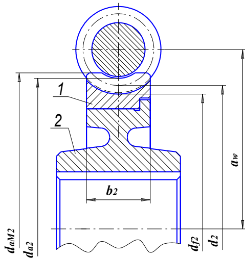
Рисунок 2 – Схема червячного колеса
