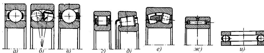
Рисунок 5.2 – Типы подшипников качения
