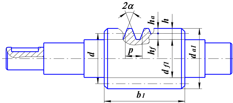
Рис. 4.1 – Червяк
