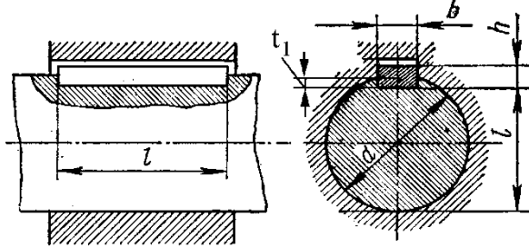
Рисунок 12 – Расчетная схема
