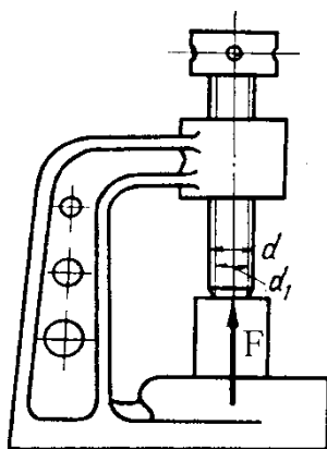
Рисунок 2 – Расчетная схема
