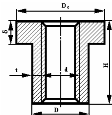
Рисунок 40 – Расчетная схема
