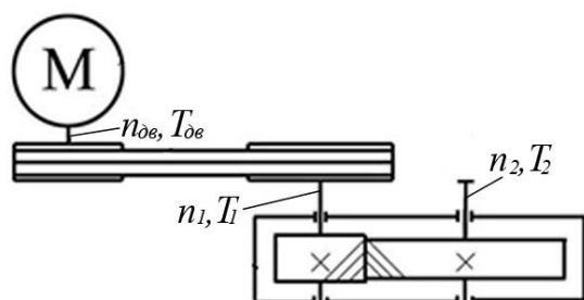
Рисунок 1 – Схема приводной станции
