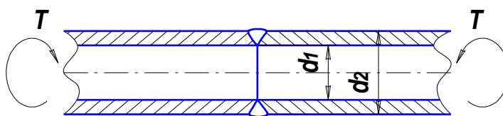
Рисунок 7.5 – Стыковое соединение труб
