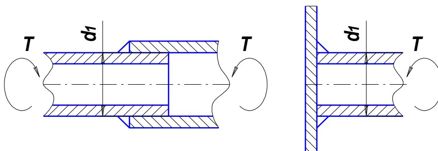
Рисунок 7.5 – Стыковое соединение труб
