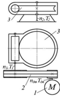
Рисунок 1 – Приводная станция:
