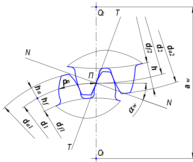
Рис. 3.1 – Зубчатое зацепление
