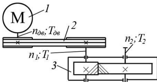
Рисунок 2.5 – Приводная станция: 1 – электродвигатель; 2 – клиноременная передача; 3 – редуктор
