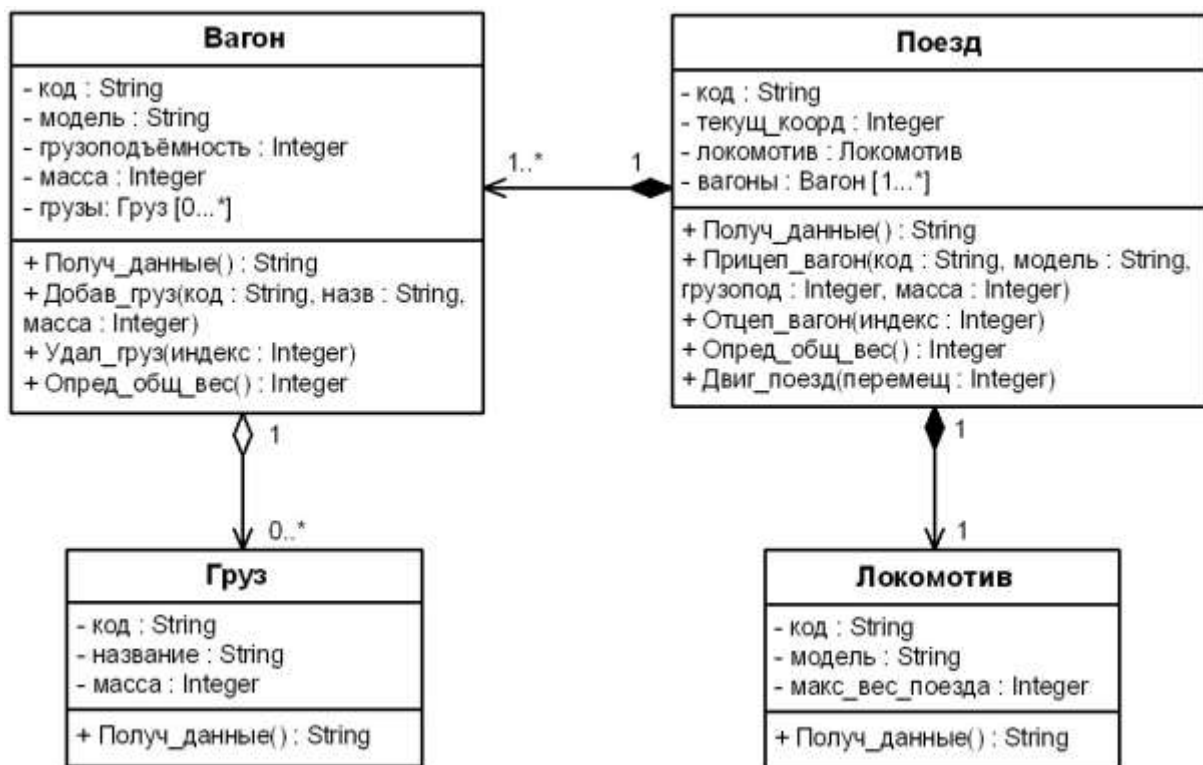
Рис. 4.1. Диаграмма классов
