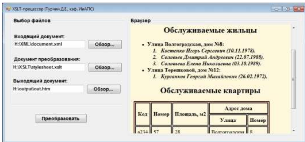
Рис. 1.8. Работа приложения
