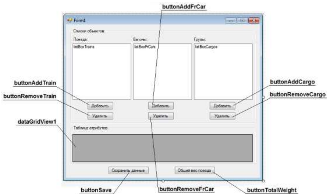
Рис. 4.12. Интерфейс пользователя
