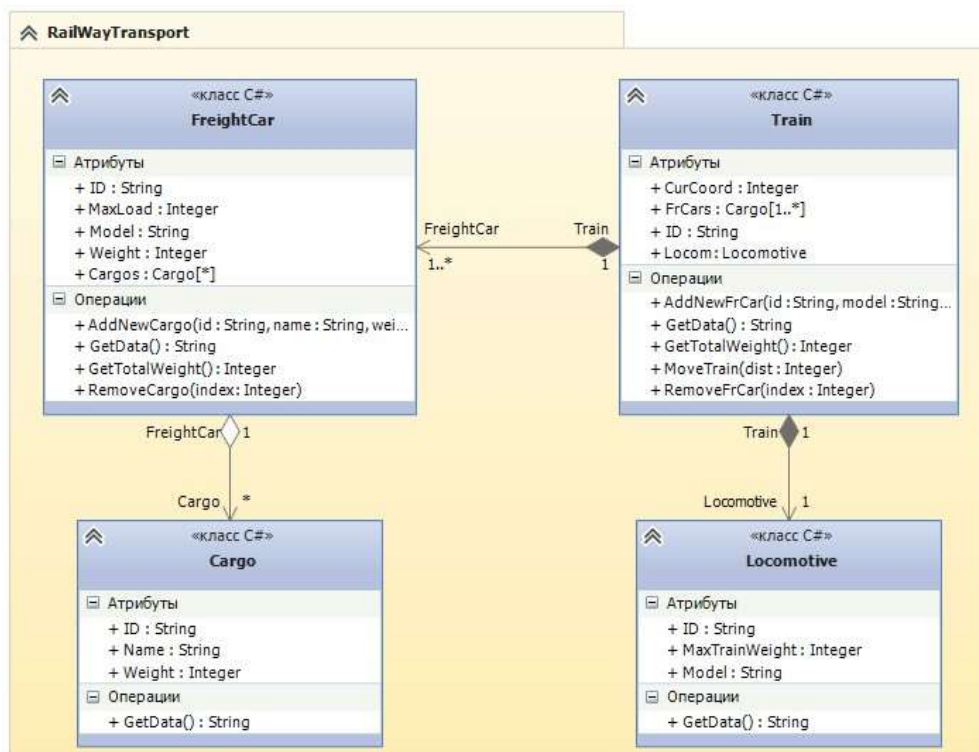
Рис. 4.10. Схема классов
