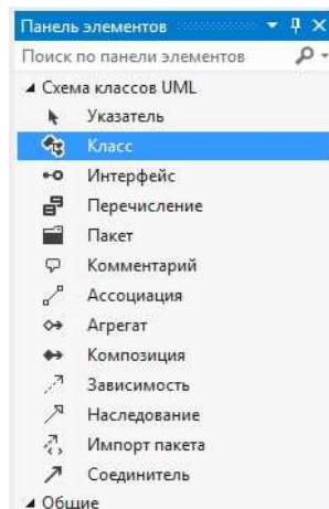
Рис. 4.5. Панель элементов
