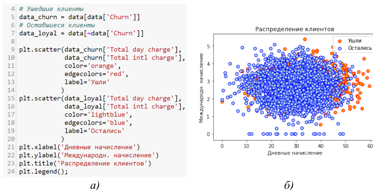
Рисунок 2.17 – Построение отдельных подмножеств с легендой; а) исходный код; б) полученный график
