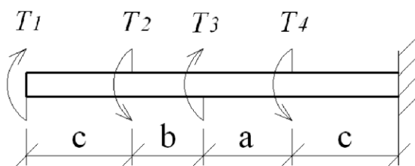
Схема вала
