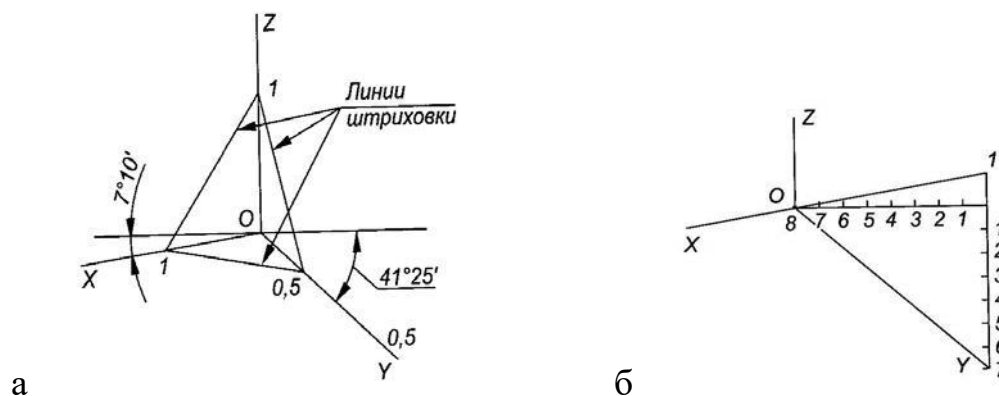
Прямоугольная диметрия. В диметрии две координатные оси одинаково наклонены к плоскости аксонометрических проекций, а третья—под другим углом. В этом случае угол между осями X и Y и горизонтальной линией равен соответственно 70^{\circ}10' и 41^{\circ}25' (рисунок 64а).
