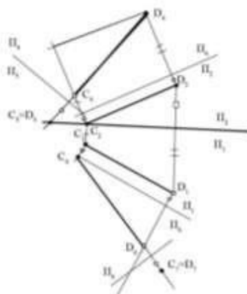
Рисунок 8.1 – Преобразования прямой
