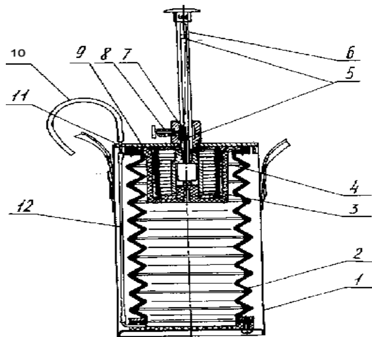
Рис. 12. Газоанализатор УГ-2
