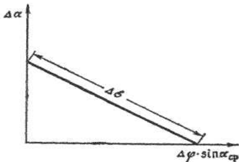
Рисунок 16 – Циркулярная номограмма
