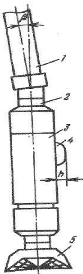
Рисунок 20 – Отклоняющее устройство с накладкой:
