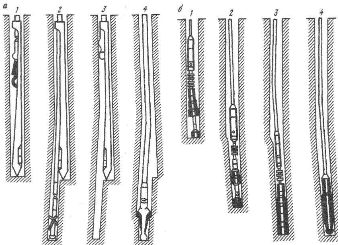
Рисунок 24 – Типы отклоняющих приспособлений в роторном бурении:
