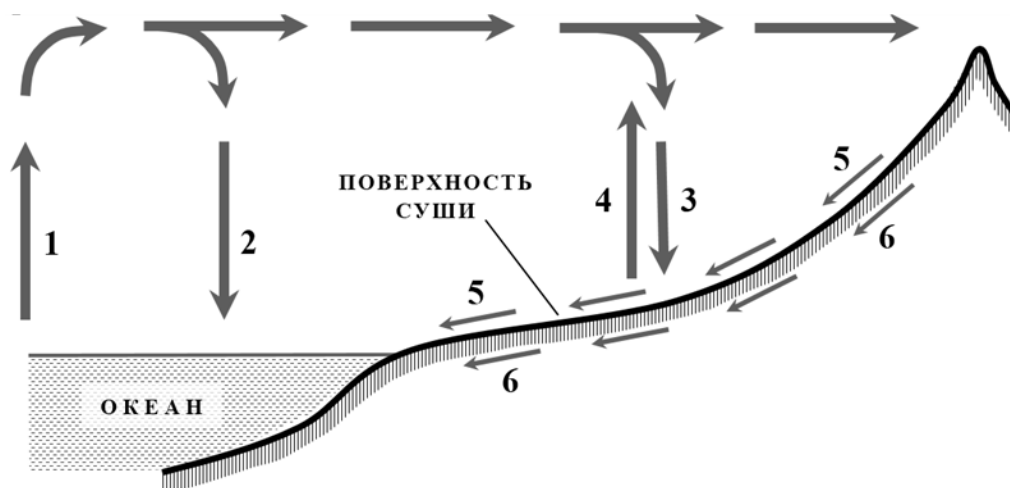
Рисунок 13. Влагооборот воды в природе
