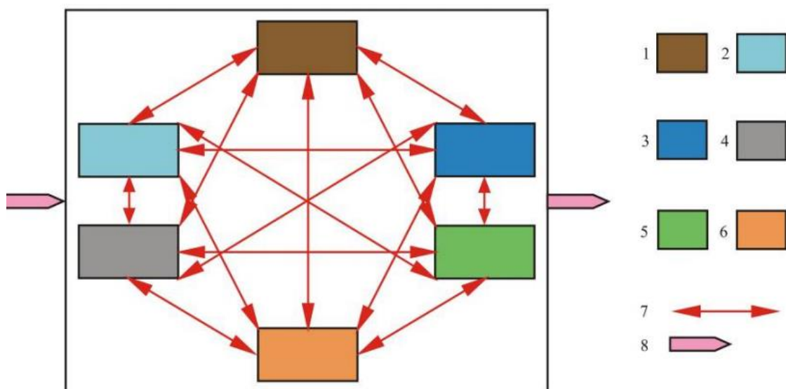
Рисунок 5. Концептуальная модель природной геосистемы
