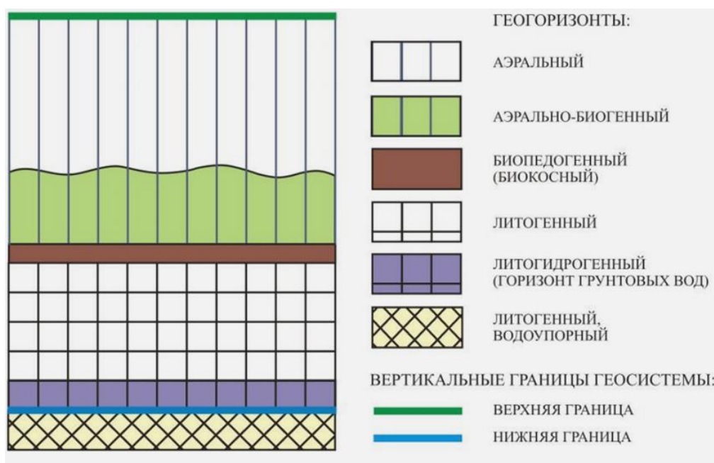
Рисунок 4. Вертикальная структура наземной природной геосистемы
