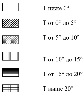
Рисунок 12. Периоды со среднесуточными температурами в определенных пределах
