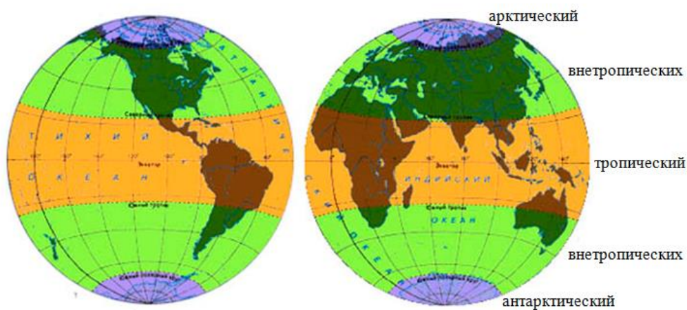
Рисунок 18. Географические пояса Земли»
