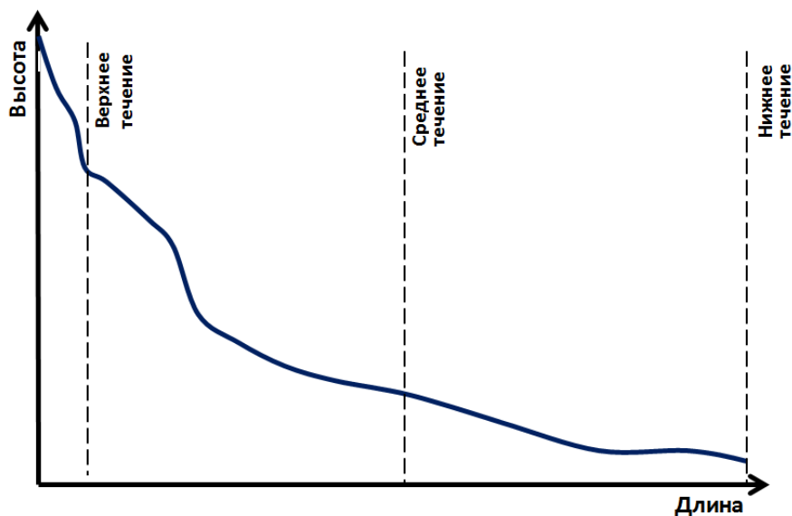
Рисунок 16. Продольный профиль реки
