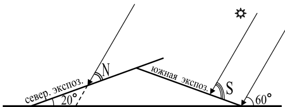
Рисунок 8. Схема распределения солнечных лучей на склонах холма
