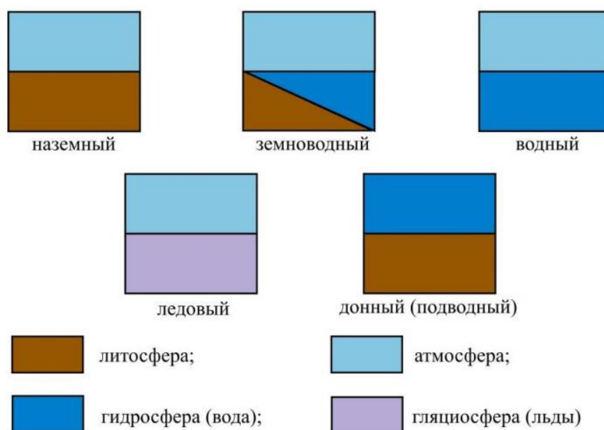
Рисунок 3. Структурные варианты ландшафтной оболочки (по Ф. Н. Милькову)
