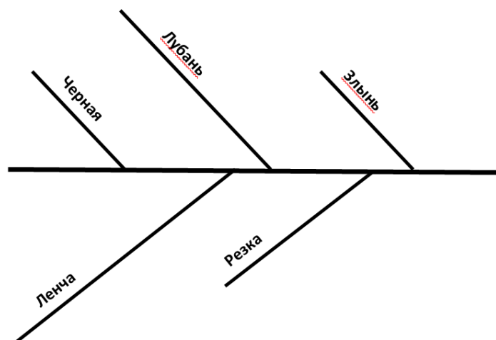
Рисунок 15. Гидрографическая схема речной системы
