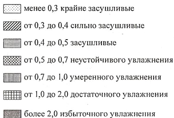
Рисунок 9. Значение коэффициента увлажнения
