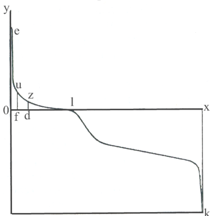
Рисунок 7. Гипсографическая кривая
