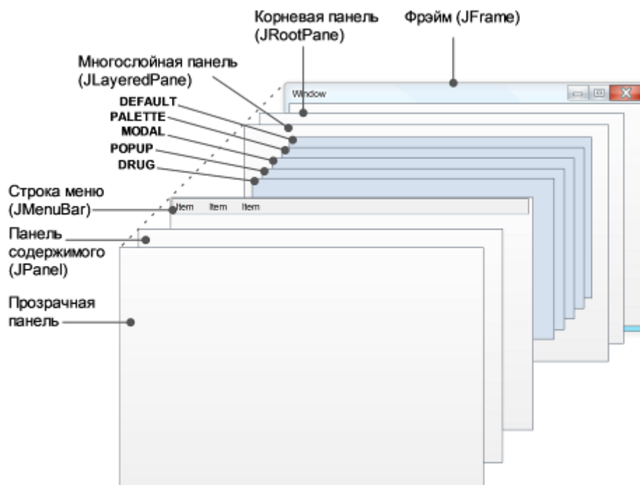
Рисунок 8.4 – Структура JFrame.
