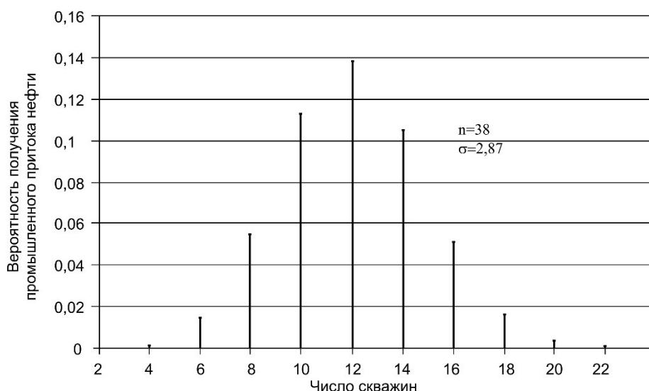
Рисунок 4.1 – Биноминальное распределение на примере изучения вероятности вскрытия нефтесодержащей части карбонатно-глинистых отложений подсвиты Морозкинской балки (нижний майкоп)
